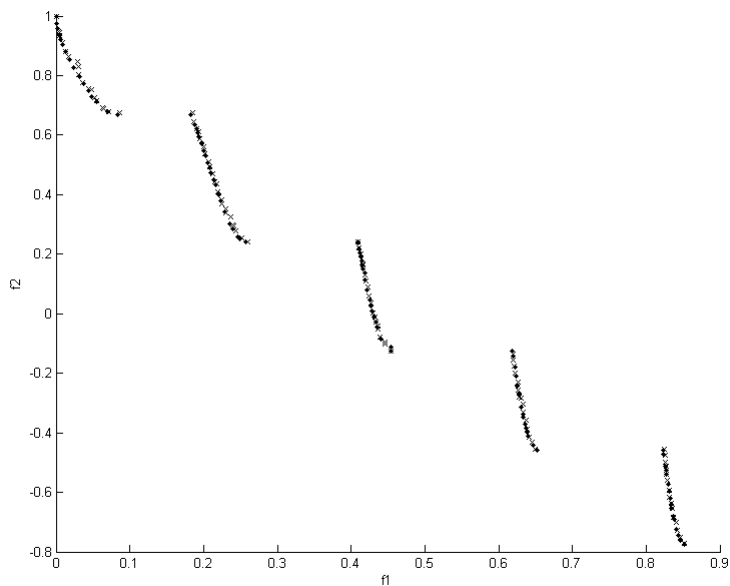
FIGURE 3.6 – Fronts de Pareto de NSGA-II et MO-TRIBES pour la fonction ZDT3. (×) Front de Pareto donné par MO-TRIBES, (.) Front de Pareto donné par NSGA-II.
