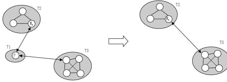
FIGURE 2.2 – Destruction de particule. La tribu T1 est détruite, les liens d'informations sont redistribués vers T2 et T3 .
