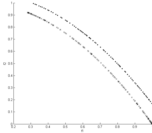
FIGURE 3.7 – Fronts de Pareto de NSGA-II et MO-TRIBES pour la fonction ZDT6. (x) Front de Pareto donné par MO-TRIBES, (.) Front de Pareto donné par NSGA-II.
