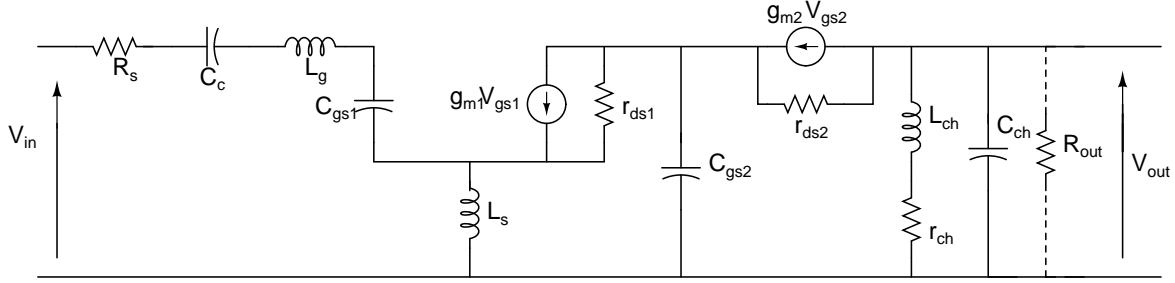
FIGURE 5.4 – Modèle petit-signal de l'amplificateur faible bruit.
