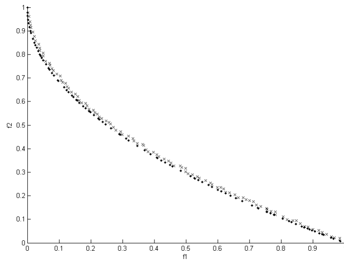
FIGURE 3.4 – Fronts de Pareto de NSGA-II et MO-TRIBES pour la fonction ZDT1. (×) Front de Pareto donné par MO-TRIBES, (.) Front de Pareto donné par NSGA-II.
