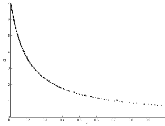
FIGURE 3.3 – Fronts de Pareto de NSGA-II et MO-TRIBES pour la fonction Deb. (×) Front de Pareto donné par MO-TRIBES, (.) Front de Pareto donné par NSGA-II.
