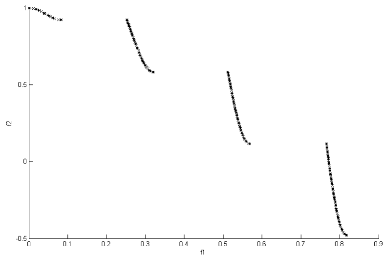
FIGURE 3.8 – Fronts de Pareto de NSGA-II et MO-TRIBES pour la fonction MOP6. (x) Front de Pareto donné par MO-TRIBES, (.) Front de Pareto donné par NSGA-II.
