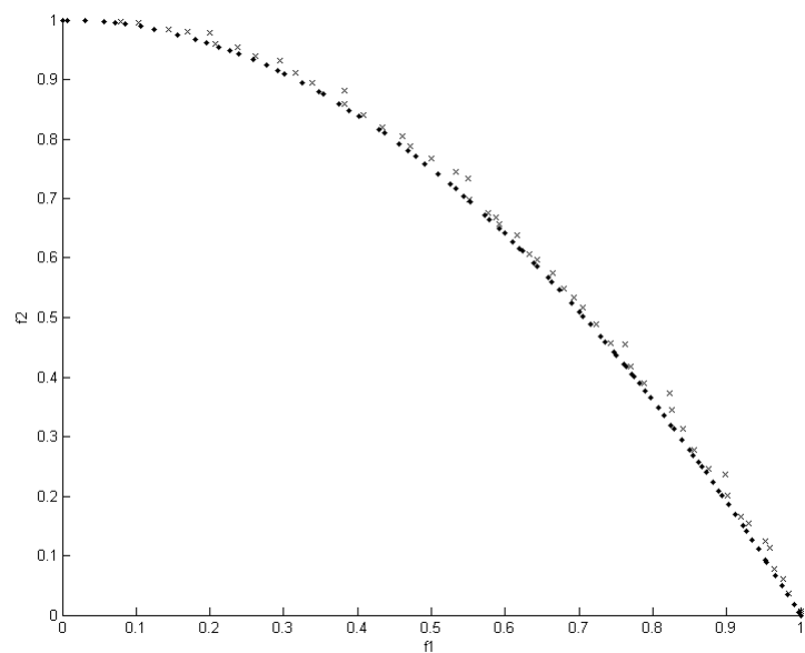
FIGURE 3.5 – Fronts de Pareto de NSGA-II et MO-TRIBES pour la fonction ZDT2. (×) Front de Pareto donné par MO-TRIBES, (.) Front de Pareto donné par NSGA-II.
