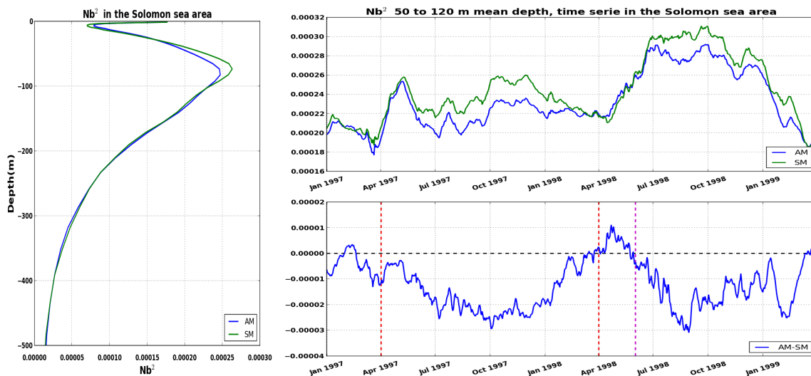
FIGURE 8.20 – Frequence de Brünt Vaisala moyennée dans la mer des Salomon pour les modèles avec marée (bleu) et sans marée (vert). A gauche, profil vertical moyen. A droite, en haut : les séries temporelles de N^2 pour les simulations AM (bleu) et SM (vert), en bas : série temporelle de l'anomalie AM-SM de N^2 . La période Niño est délimitée par les lignes verticales pointillées rouge, la période Niña se situe à droite de la ligne en magenta
