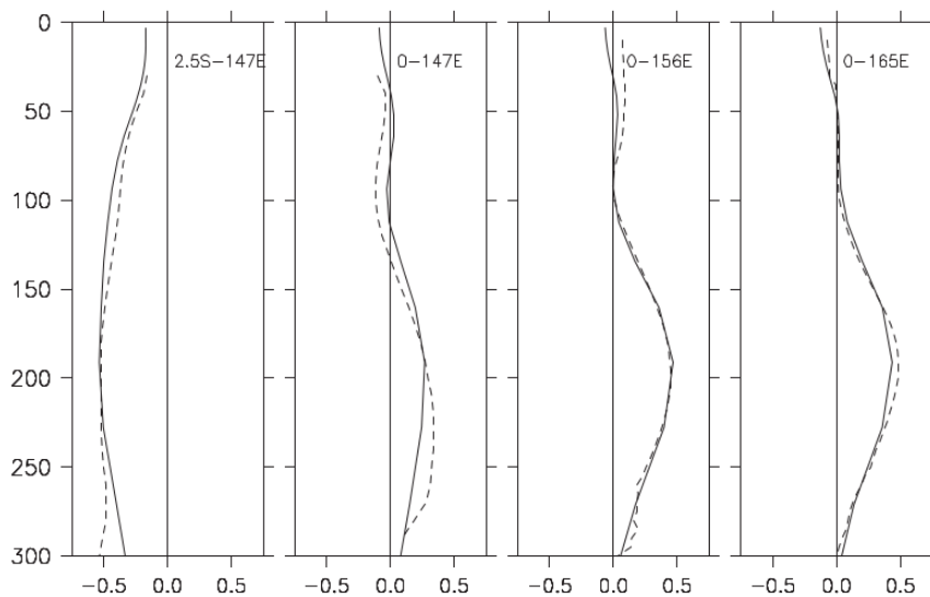
FIGURE 5.2 – Comparaison de profil vertical de courant moyen 1978-2011 entre le modèle au 1/12° et les observations TAO. Source :Gourdeau et al. (2014)
