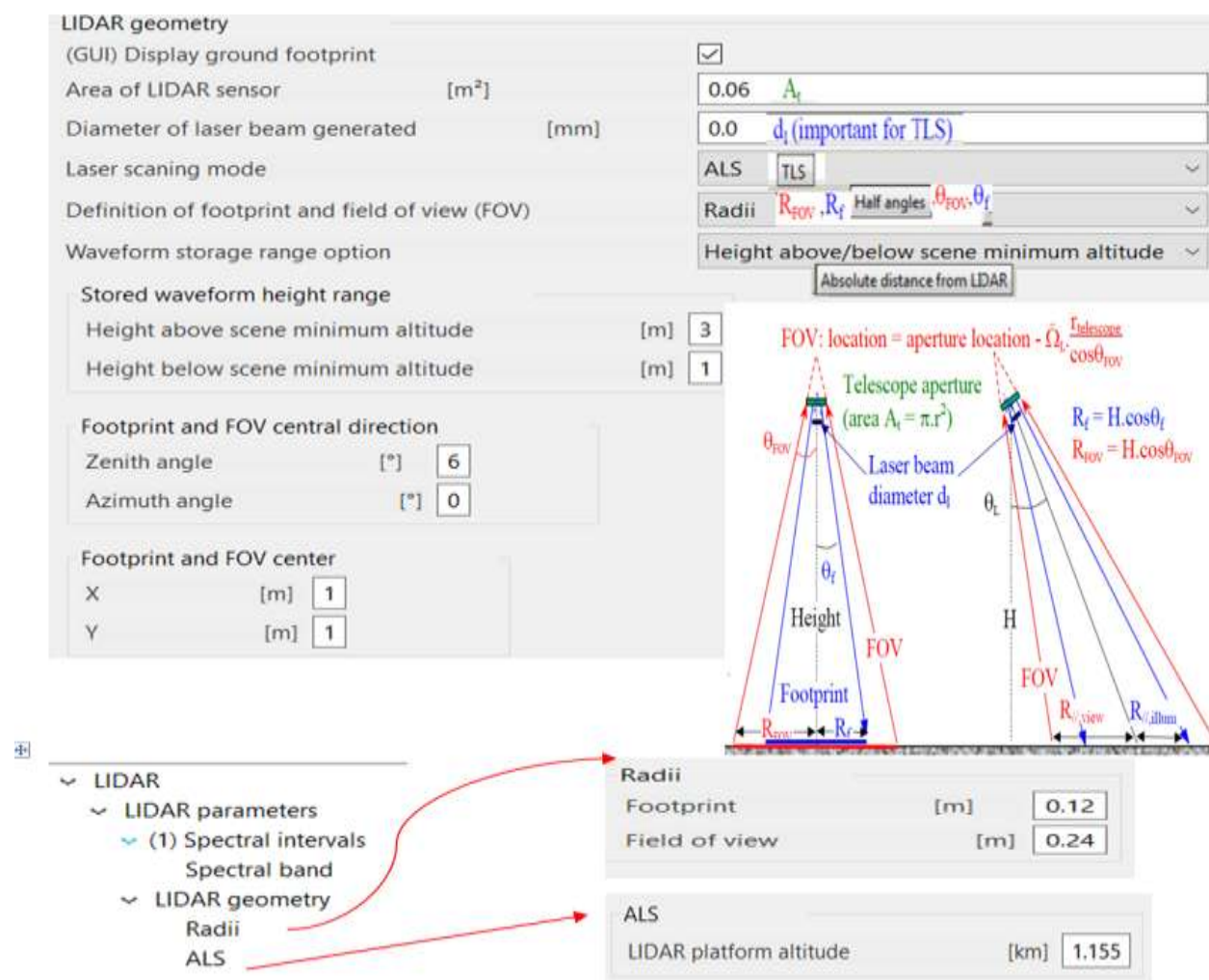
Figure 1-16 : Paramètres de la géométrie du LiDAR ALS en mode "simple pulse" dans DART.
