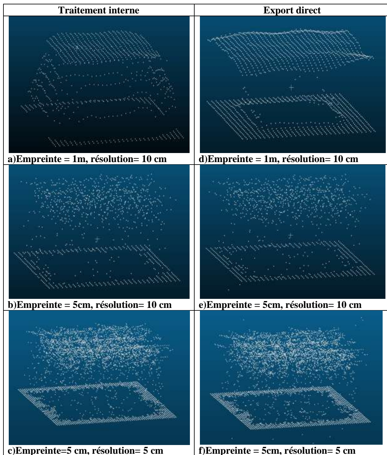
Figure 1-27 : Affichage des nuages de points générés par le module de décomposition gaussien avec ses deux types « traitement interne » (a, b, c) et « export direct » (d, e, f) traités par l'outil Cloud Compare.
