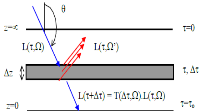
Figure 1-3: Altitude z et épaisseur optique \tau au sein d'une couche plane homogène. Ici, l'épaisseur optique au sommet de la couche est nulle. Pour tout trajet dr(\Omega) = \frac{dz}{\cos\theta} , d\tau \cdot \cos\theta < 0 . \cos\theta est souvent noté \mu .
