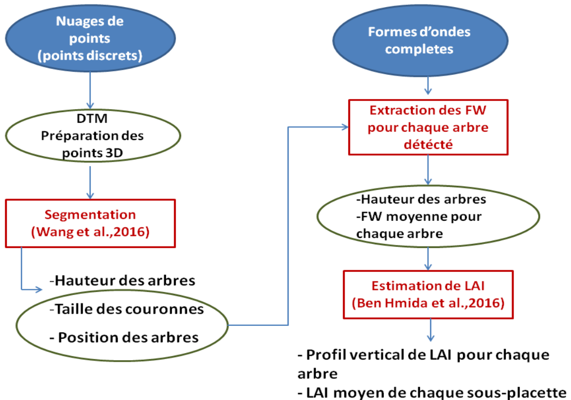
Figure 4-4 : Diagramme schématisé de la méthodologie d'inversion des données LiDAR réelles pour l'estimation des propriétés des forêts.
