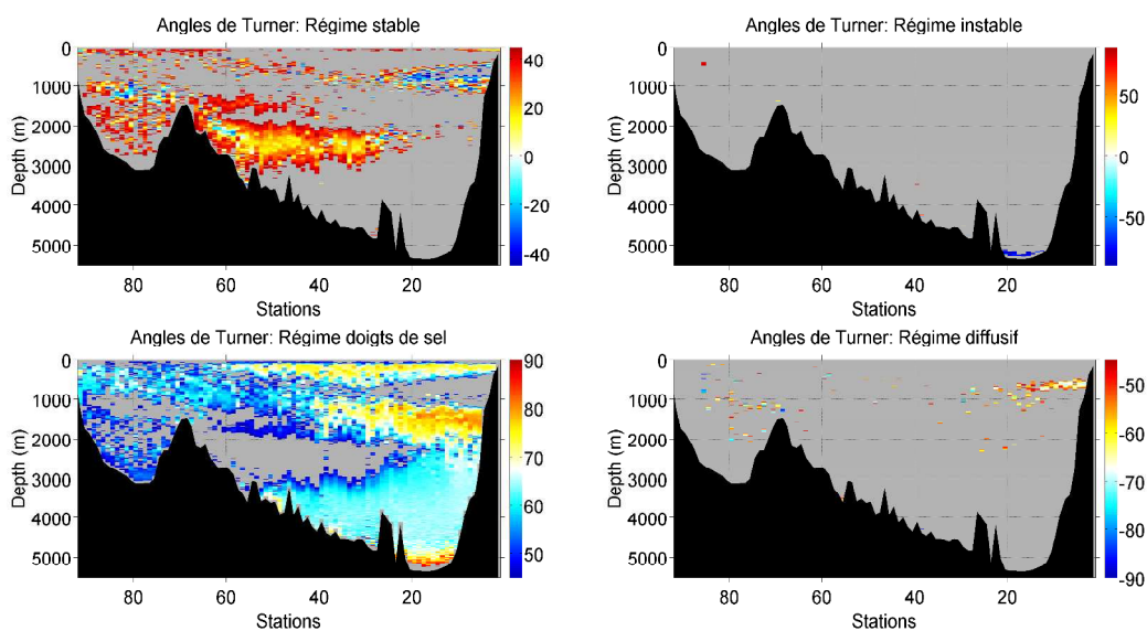
FIGURE 5.24 – Ovide 2008. Angles de Turner pour les différents régimes possibles de stabilité de la colonne d'eau. Les échelles de couleur sont différentes pour chacun de régimes.
