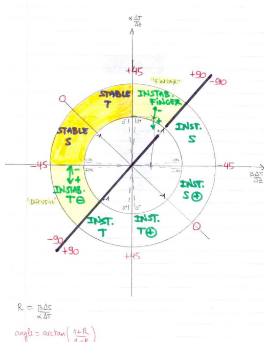
FIGURE 5.23 – Cadran des angles de Turner.
