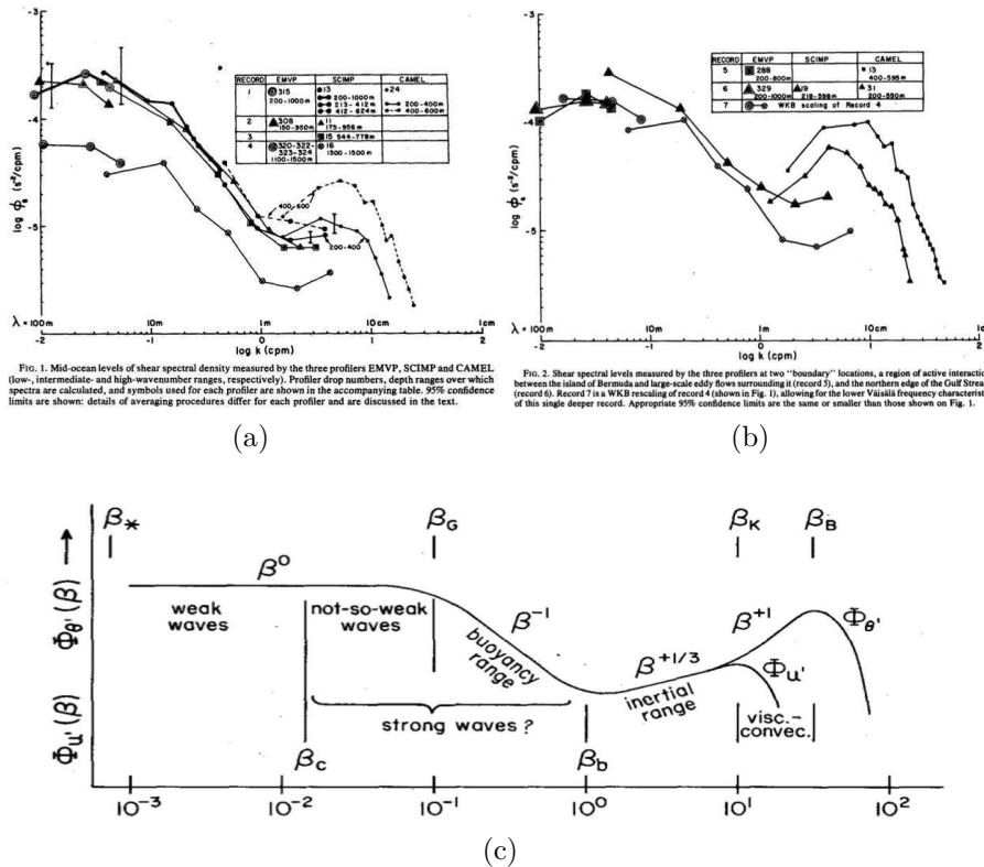
FIGURE 2.10 – (a et b) Spectre composite du cisaillement vertical des vitesses horizontales (shear), construit à partir de différents jeux de mesures (figure tirée de Gargett et al. (1981)). (c) Spectre schématique du cisaillement vertical des vitesses horizontales et du gradient de température. Le nombre d'onde vertical \beta est ici exprimé en cycle/m . Le spectre est plat, en \beta^0 , dans le domaine ondulatoire, pour des longueurs d'ondes allant de plusieurs centaines de mètres jusqu'à 10m. Le domaine de fine-structure est caractérisé par la pente en \beta^{-1} , entre 10 et 1m. En dessous on accède au domaine de la micro-structure, de l'ordre du mètre jusqu'au millimètre, où les termes dissipatifs deviennent significatifs (figure tirée de Holloway (1983)).
