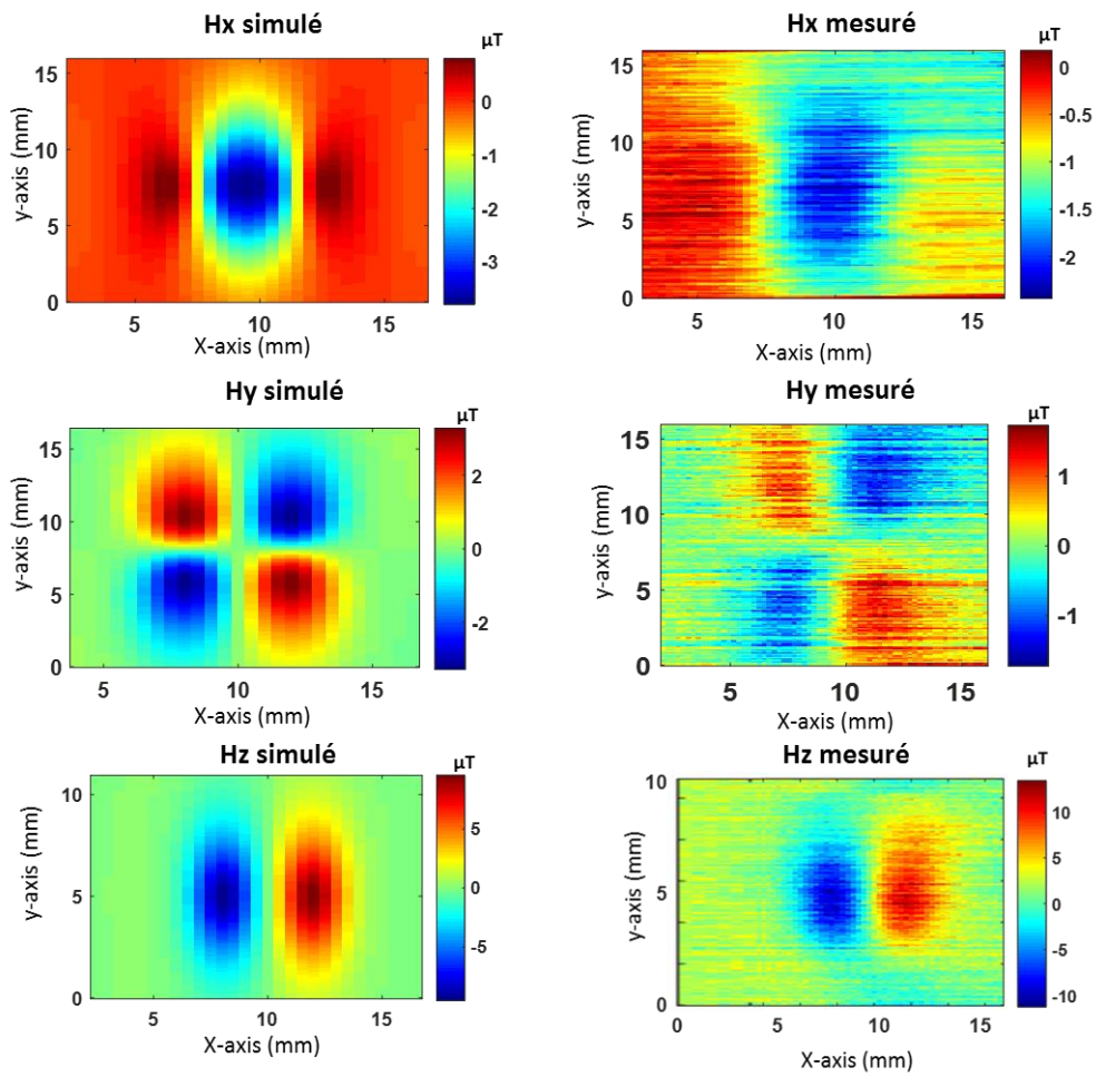
Figure 5 : Résultats de simulation ( partie gauche ) et résultats expérimentaux ( partie droite )
