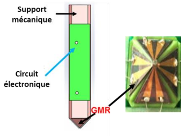
Figure 1 : vue schématique de la sonde ( partie gauche ) photo de la tête de la sonde montrant les 4 triangles de silicium comportant au bout un élément GMR en forme de C ( partie droite )
