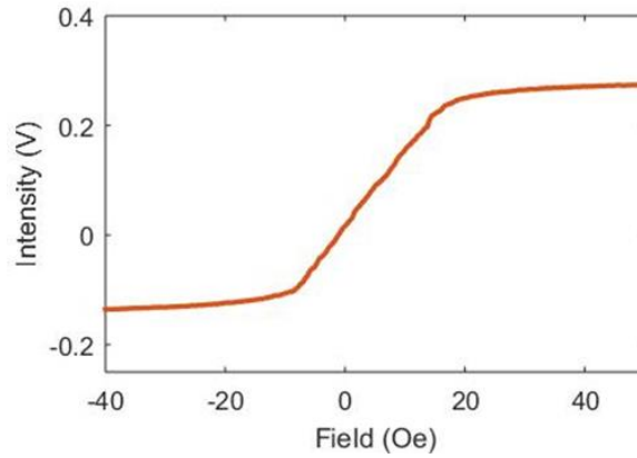
Figure 2 : exemple de réponse d'une GMR en fonction du champ magnétique appliqué le long de son axe de sensibilité
