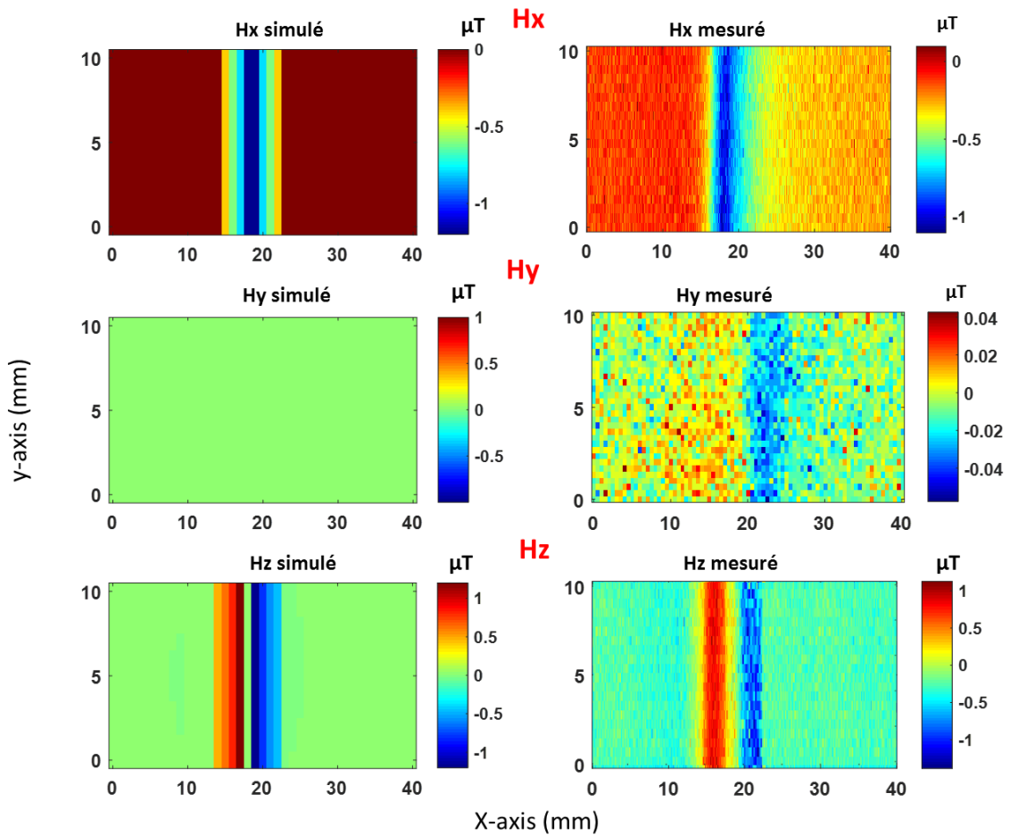
Figure 4 : balayage 2D du champ magnétique d'une ligne de courant excitée par un courant continu de 20 mA; Résultats des trois composantes simulés ( partie gauche ) et les trois composantes du champ mesurés par la sonde 3D ( partie droite ).
