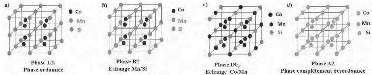
Figure1: présentation schématique des quatre phases cristalline pour le Co 2 MnSi a) L 21 , b) B2, c) D0 3 et A2.
