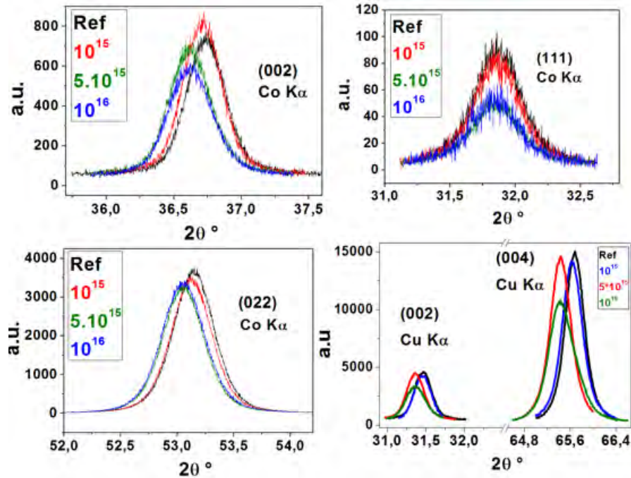
Figure 6: Diffraction des rayons X . 2\theta scan pour l'échantillon de référence et les 3 échantillons irradiés pour les sources de Co et Cu. a), b) et c) représente les 111,002 et 022 pics acquis avec la source de Co. d) et e) présente les pics 002 et 004 acquis avec la source de Cu.
