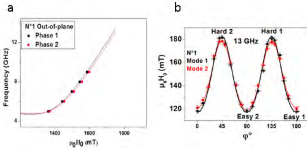
Figure 15: relation de dispersion pour l'échantillon de référence pour un champ appliqué perpendiculairement au plan de la couche. b) dépendance angulaire du champ de résonance à 13 GHz pour un champ appliqué dans le plan de la couche.
