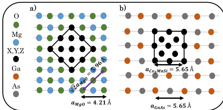
Figure 2: e présentation schématique de la croissance épitaxial du Co 2 MnSi sur a) MgO et b) GaAs.
