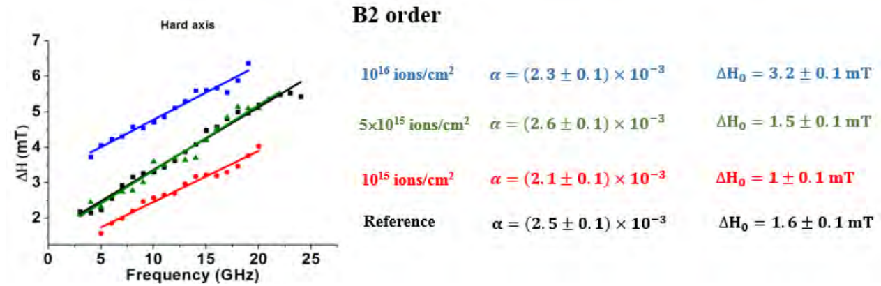
Figure 24: Evolution avec la fluence de la largeur de raie pour la phase B2 pour un champ appliqué dans une direction de difficile aimantation.
