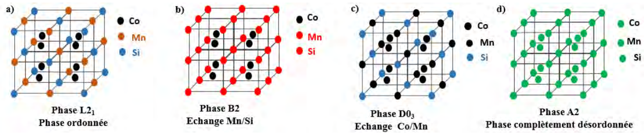
Figure1: présentation schématique des quatre phases cristalline pour le Co 2 MnSi a) L 21 , b) B2, c) D0 3 et A2.
