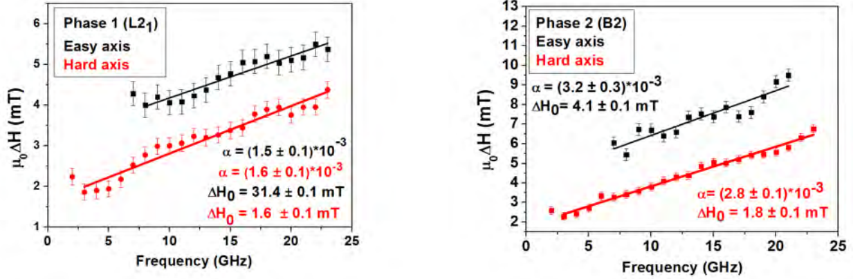
Figure 22 : Largeur de raie en fonction de la fréquence pour un champ appliqué le long des axes faciles et difficiles pour les deux phases observée L2 1 (gauche) et B2 (droite) pour l'échantillon de référence.
