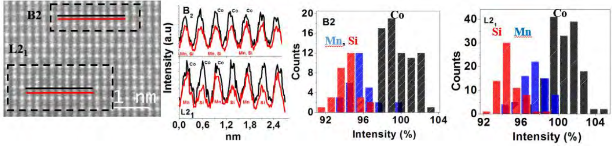
Figure 10: Image STEM-HAADF sur l'échantillon irradié à 1016 ions/cm². Les statistiques ont été effectuées sur les colonnes atomiques délimitées par les zones entourées en a).
