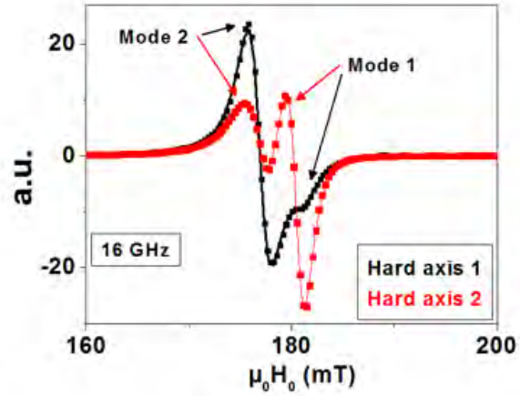
Figure 13: Les spectres d'absorption à 16 GHz en fonction du champ externe à deux axes durs.
