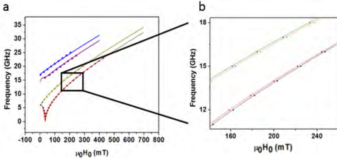
Figure 14: a) relation de dispersion F_{\text{res}} vs. \mu_0 H_0 pour l'échantillon de référence pour un champ appliqué dans le plan de la couche. A droite, zoom sur les deux modes délimités par la boîte noire en a).
