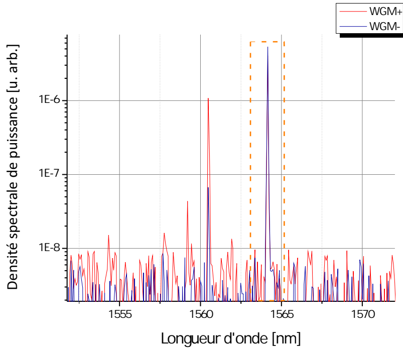
FIGURE 6.5 – Spectres optiques des signaux WGM+ et WGM- mesur s   l'OSA.
