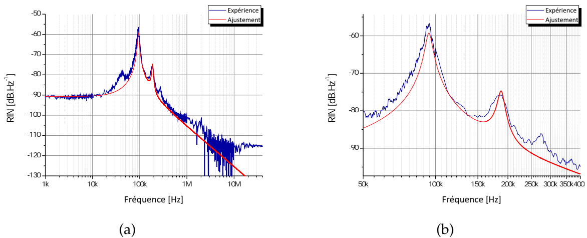
FIGURE 5.17 – RIN d'un laser WGM couplé par taper, pompe multimode : (a) spectre expérimental et ajustement théorique, (b) zoom autour de la fréquence de relaxation.
