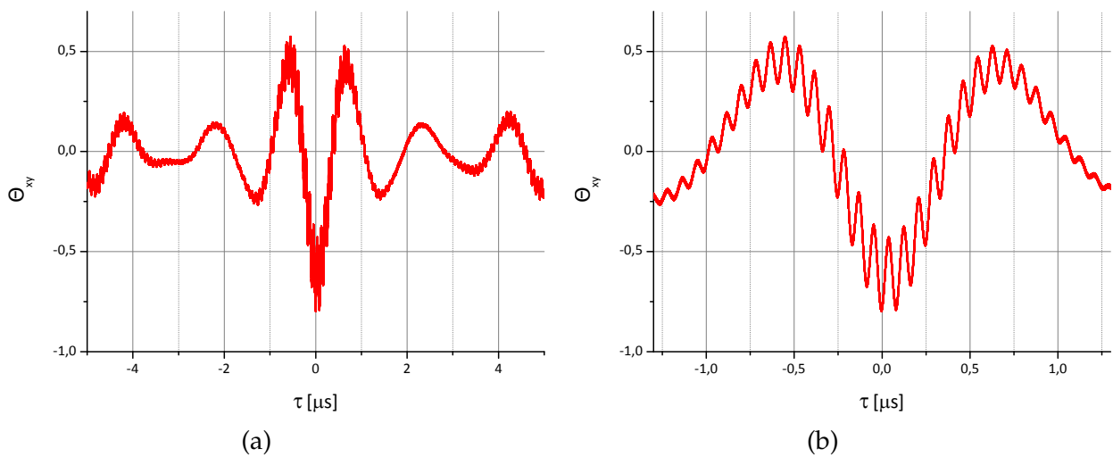
FIGURE 6.8 – (a) Fonction d'intercorrélation normalisée \Theta_{xy} des signaux photodétectés réduits, G = 10^5 \text{ V}\cdot\text{A}^{-1} , (b) zoom autour de \tau = 0 .
