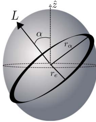
FIGURE 2.4 – Représentation d’un ellipsoïde de révolution d’axe \mathbf{u}_z de type prolata. Le champ électromagnétique circulant dans ce résonateur est caractérisé par son moment angulaire \mathbf{L} et décrit une trajectoire elliptique d’axes r_e et r_\alpha . \mathbf{L} précesse’ autour de l’axe \mathbf{u}_z avec un angle \alpha = \arccos(L_z/L) .
