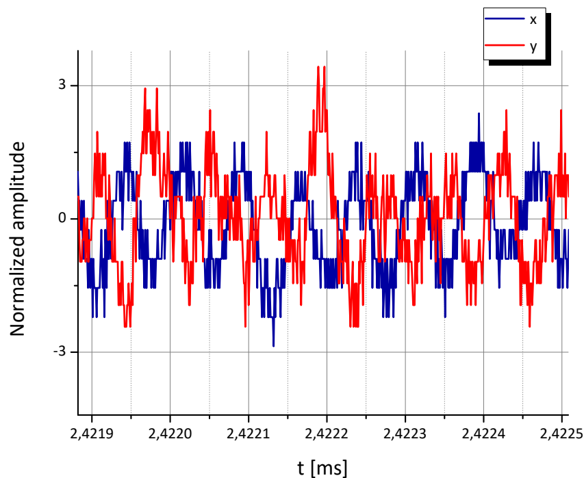
FIGURE 6.7 – Traces temporelles des tensions réduites x et y dans un micro-résonateur en IOG-1, G = 10^5 \text{ V}\cdot\text{A}^{-1} .
