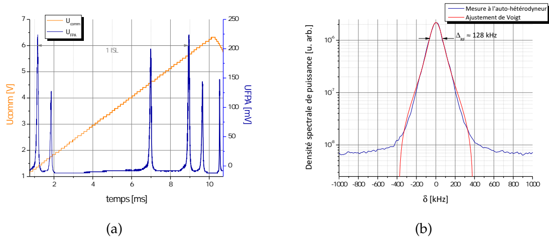
FIGURE 5.12 – (a) Spectre optique d'un laser WGM multimode mesuré au Fabry-Perot d'analyse (b) Largeur de raie mesurée à l'auto-hétérodyneur dans le domaine électrique ( \delta est le désaccord à la fréquence de modulation du modulateur acousto-optique).
