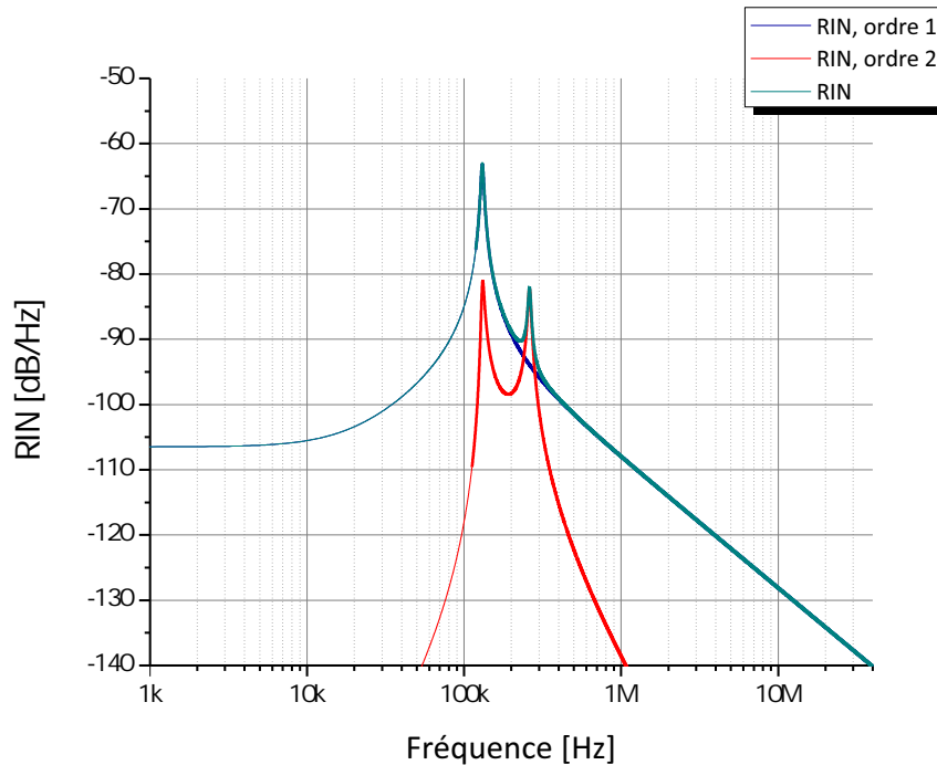
FIGURE 5.7 – Spectre du RIN théorique d'un laser de classe B dopé Erbium pour r = 2 , \tau_p = 150 \text{ ns} , T_1 = 10 \text{ ms} , \kappa = 0.025 \text{ s}^{-1} ( \mathcal{V} \simeq 2400 \text{ } \mu\text{m}^3 ), D_{NN} = 10^{17} \text{ s}^{-1} et D_{FF} = 10^{14} \text{ s}^{-1} développé jusqu'à l'ordre 2.
