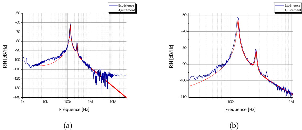
FIGURE 5.16 – RIN d'un laser WGM en Er : ZBLALiP couplé par taper droit, pompage monomode : (a) spectre expérimental et ajustement théorique, (b) zoom autour de la fréquence de relaxation.
