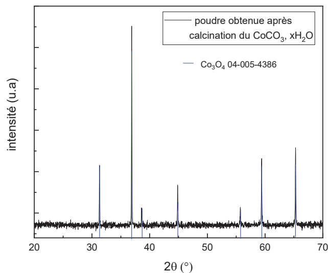
Figure 2-3 : Diffractogramme obtenu après traitement thermique de CoCO 3 ·xH 2 O à 900°C pendant 10h ; les lignes verticales bleues correspondent aux pics donnés dans la fiche JCPDS 04-005-4386 du Co 3 O 4 .
