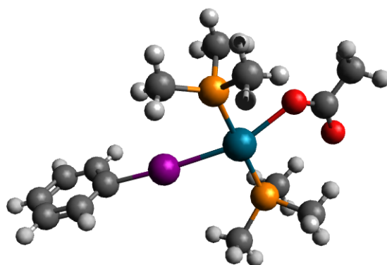
FIGURE II.4 – Complexe de palladium(0) anionique PhI-Pd(PMe 3 ) 2 (AcO) - calculé par GOOSSEN et coll. mettant en évidence une pseudo-liaison halogène Pd-I-C. 20
