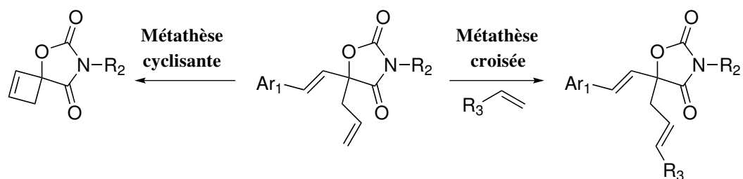
SCHÉMA III.57 – Métathèses envisageables sur l'oxazolidine-2,4-dione formée.
