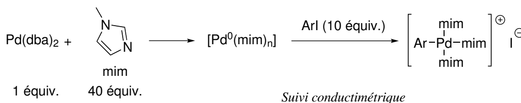
SCHÉMA II.27 – Expérience générique réalisée pour le suivi conductimétrique de l'addition oxydante de Pd 0 (mim) n sur ArI.
