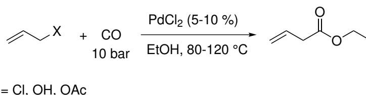
SCHÉMA III.4 – Carbonylation catalytique de dérivés allyliques catalysée par PdCl 2 , décrite par TSUJI et coll. 5
