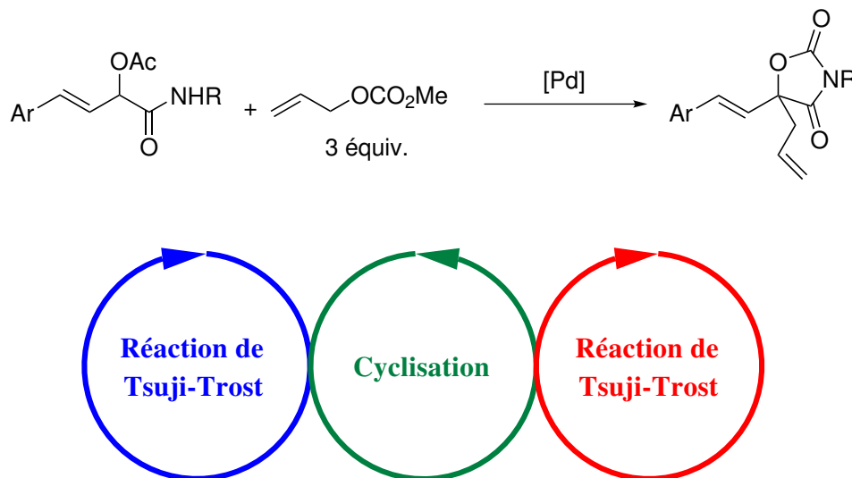
SCHÉMA III.59 – Synthèse d'oxazolidine-2,4-diones par double réaction de TSUJI-TROST et cyclisation à partir d'adduits de PASSERINI et d'allylméthylcarbonate.
