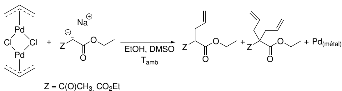
SCHÉMA III.2 – Substitution nucléophile sur le dimère [\text{Pd}(\eta^3\text{-C}_3\text{H}_5)\text{Cl}]_2 rapportée par TSUJI et coll. 3
