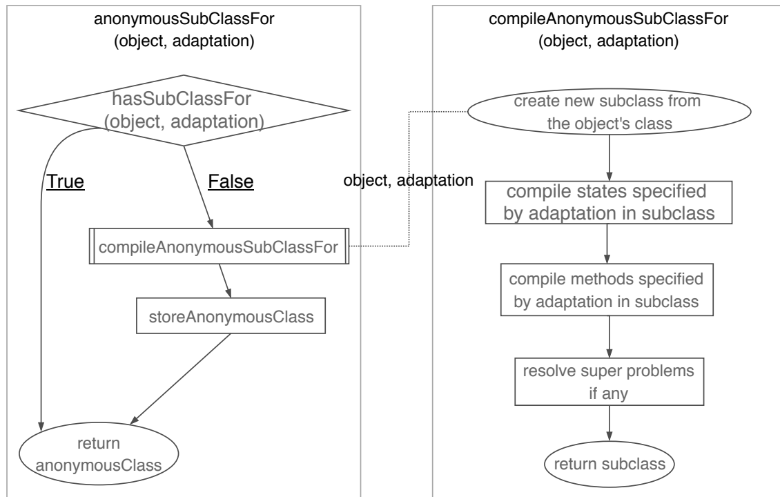
FIGURE 4.7 – Algorithme de génération de sous-classe anonyme pour un couple \{objet, adaptation\} . L'interface publique pour demander la génération d'une classe est la méthode publique anonymousSubClassFor .
