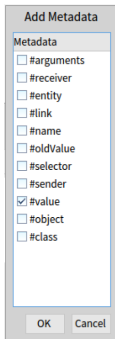
FIGURE 5.11 – Sélection des réifications primitives fournies par Reflectivity. La liste de réifications disponibles peut varier selon le type de nœud ciblé par les points de collecte.
