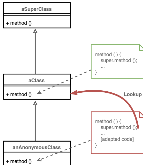
FIGURE 4.3 – Problème du super , dû à la mise en œuvre par sous-classes anonymes. Le lookup pour les envois de message à la pseudo-variable super est démarré dans la classe d'origine du receveur ( aClass ) au lieu de démarrer dans la super classe de cette dernière ( aSuperClass ).
