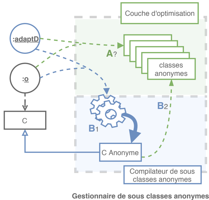
FIGURE 4.6 – Le gestionnaire prend en entrée une adaptation et un objet pour générer une classe anonyme. Si une classe correspondant exactement à l’adaptation pour l’objet spécifié a déjà été générée, elle est retournée immédiatement (A). Sinon, la sous-classe est générée à partir de la classe de l’objet, puis les modifications de comportement spécifiées par l’adaptation sont compilées dans cette sous-classe ( B_1 ). Enfin, la sous-classe est stockée par la couche d’optimisation ( B_2 ) avant d’être retournée.
