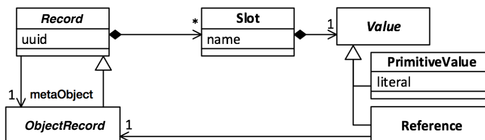
FIGURE 3.3 – Modèle d'exécution minimal
