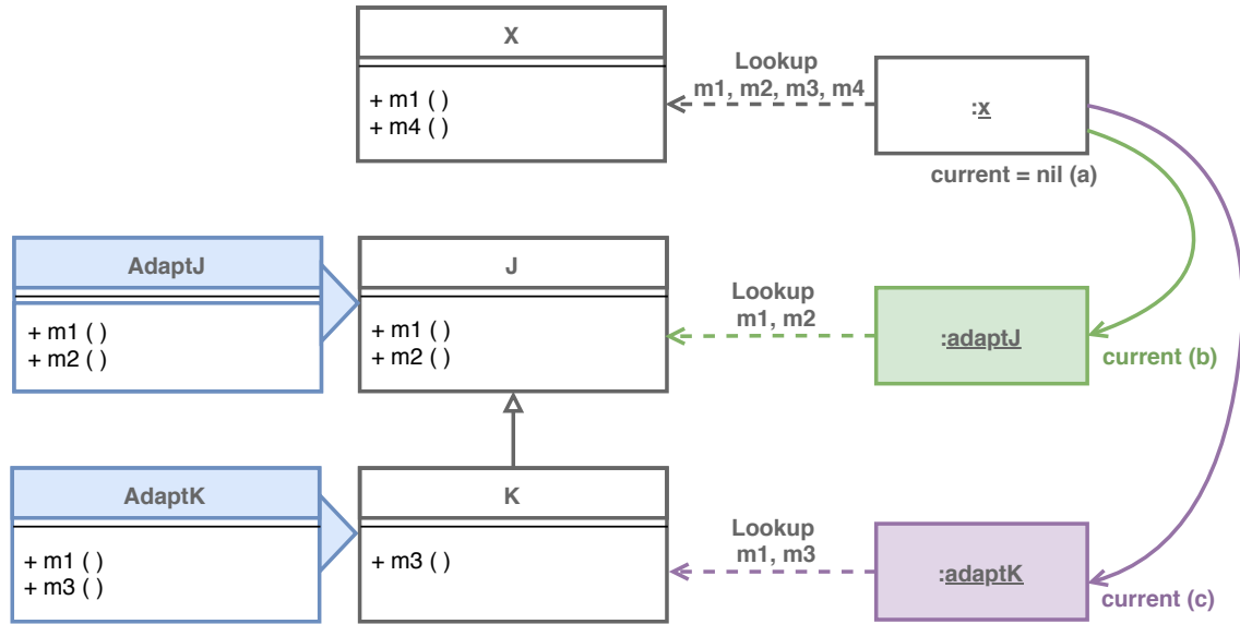
FIGURE 3.8 – (a) x n'est pas adapté, son lookup démarre dans son méta-objet (sa classe). (b) x est adapté par une instance de LUBRecord adaptJ , instance de l'adaptation AdaptJ . Le lookup pour les méthodes sélectionnées ( m1 , m2 ) démarre alors dans la classe cible de l'adaptation ( J ). Le lookup pour les méthodes non adaptées démarre dans le méta-objet d'origine de x . (c) Une nouvelle adaptation adaptK est associée à x pour les méthodes m1 , m3 . Le lookup pour m1 , m3 démarre désormais dans K tandis que pour les méthodes non adaptées ( m2 , m4 ), le lookup démarre dans X .
