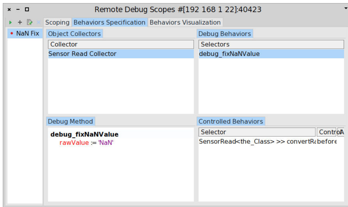
FIGURE 6.6 – La spécification d'adaptation pour un collecteur. Chaque adaptation contient un ensemble de méthodes définies par l'utilisateur-riche ainsi qu'un contrôle, qui spécifie comment une méthode adaptée s'insère dans le comportement d'un objet. Chaque collecteur possède sa propre adaptation, définie par l'ensemble des méthodes et des contrôles définis dans cette interface.
