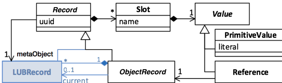
FIGURE 3.6 – Modèle d'exécution de Lub étendu avec Adaptation
