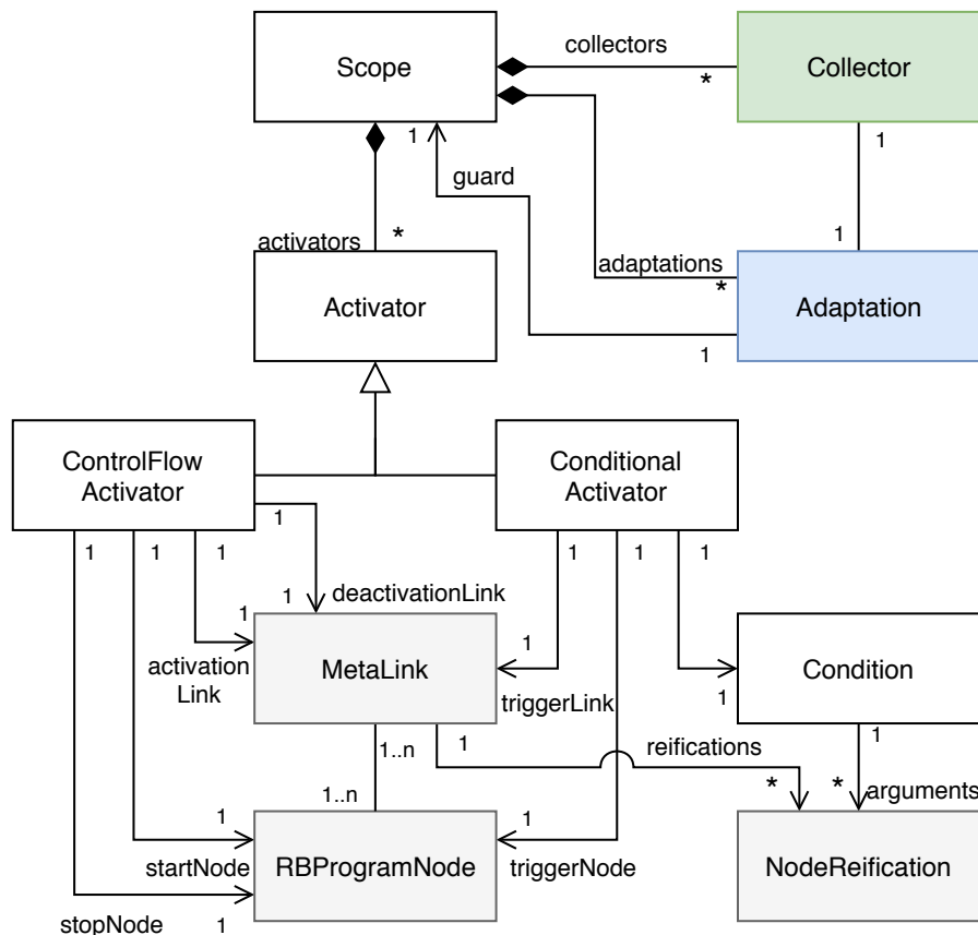
FIGURE 6.2 – Modèle de mise en œuvre des Debug-Scope .
