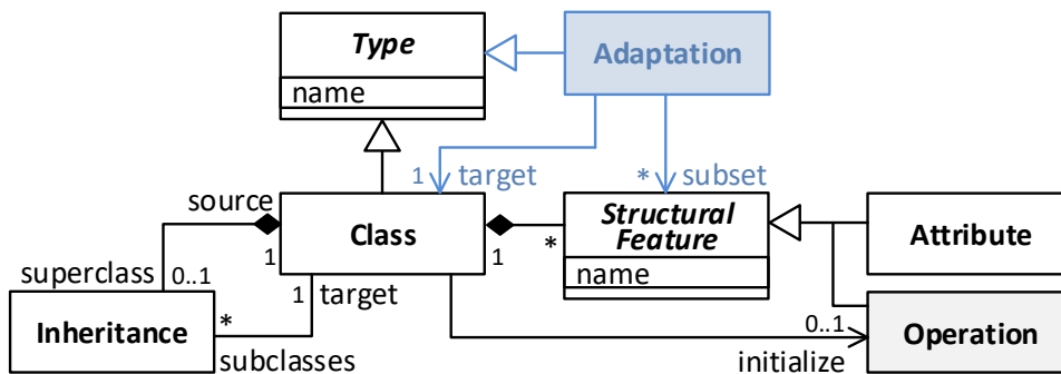
FIGURE 3.4 – Infrastructure de Lub : Kernel-Lub étendu avec Adaptation
