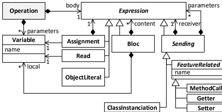
FIGURE 3.2 – Opérations du langage minimal
