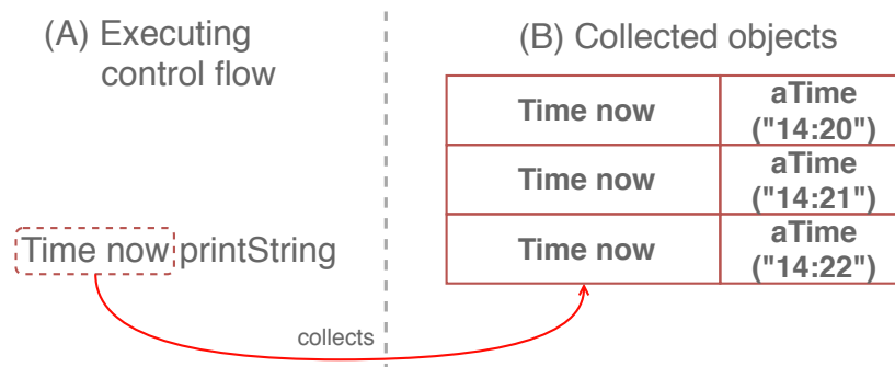
FIGURE 3.12 – Illustration d'un collecteur : le collectPoint est une expression particulière du programme Time now (A), dont le résultat de l'évaluation sera collecté et stocké par le collecteur (B).
