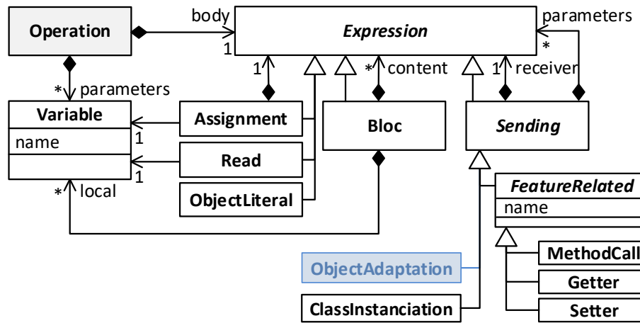
FIGURE 3.5 – Opérateurs de Lub étendus avec Adaptation
