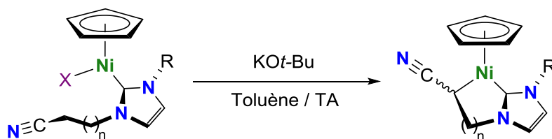
Schéma 2. Synthèse de nickelacycles par activation d'une liaison C–H en \alpha d'un groupement nitrile.
