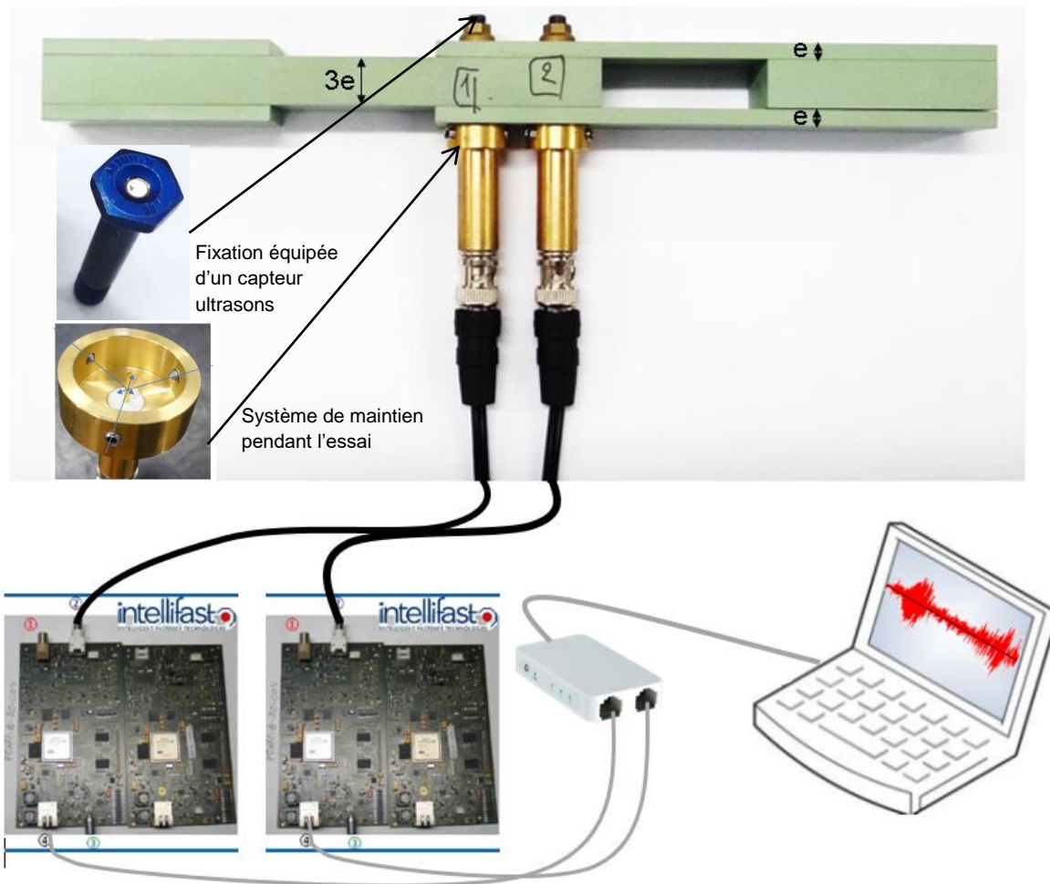
Figure 4. 26 : Eléments composant le système de suivi dynamique de prétension
