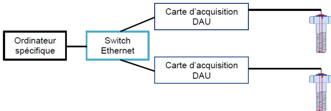
Figure 4. 25 : Architecture du moyen de suivi dynamique de précontrainte
