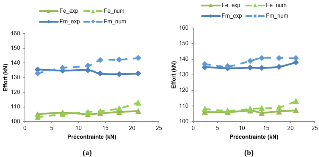
Figure 5. 8 : Comparaison entre le comportement statique numérique et expérimental pour un assemblage en double cisaillement ajusté (a) et avec interférence de -50µm (b)
