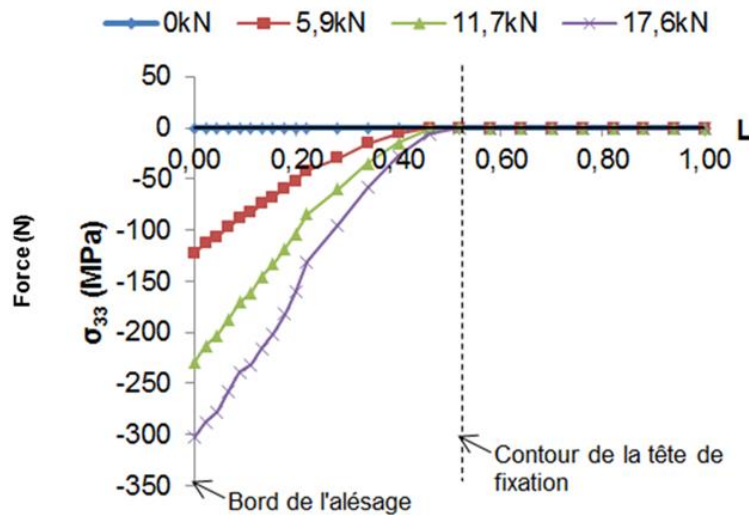
Figure 2. 19 : Evolution des contraintes \sigma_{33} suivant le chemin PT s en fonction de la précontrainte pour un chargement de 100MPa sur la section nette
