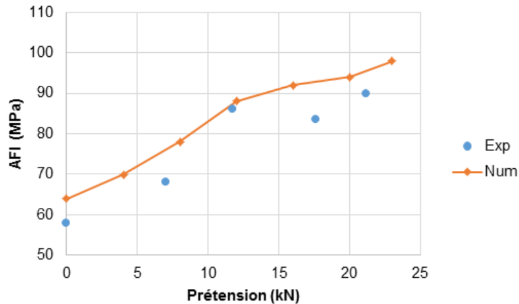
Figure 5.21 : Effet de la précharge sur l'AFI
