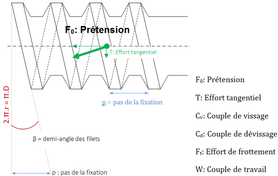
Figure A2. 1 : Notations utilisées
