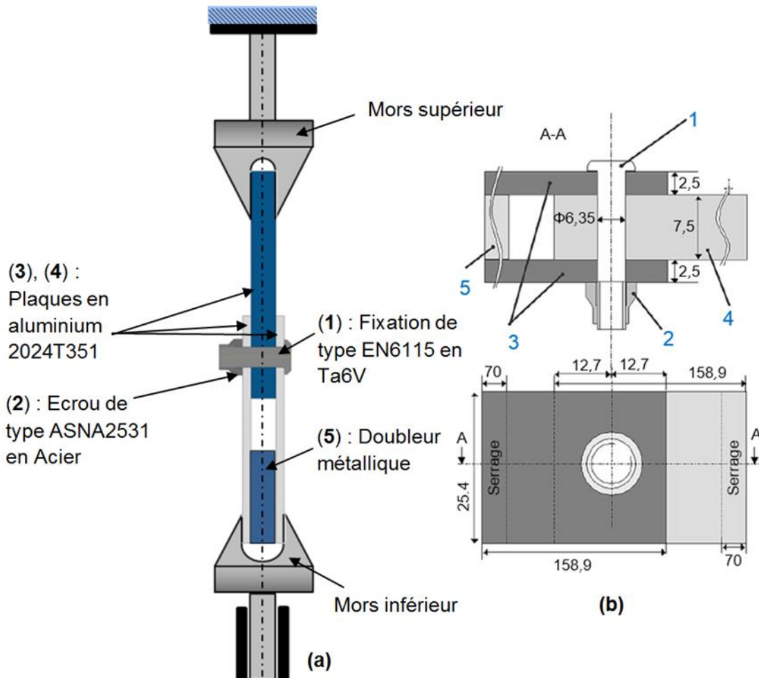
Figure 2. 1 : (a) Type de chargements considérés (b) Dimensions de l'assemblage de référence
