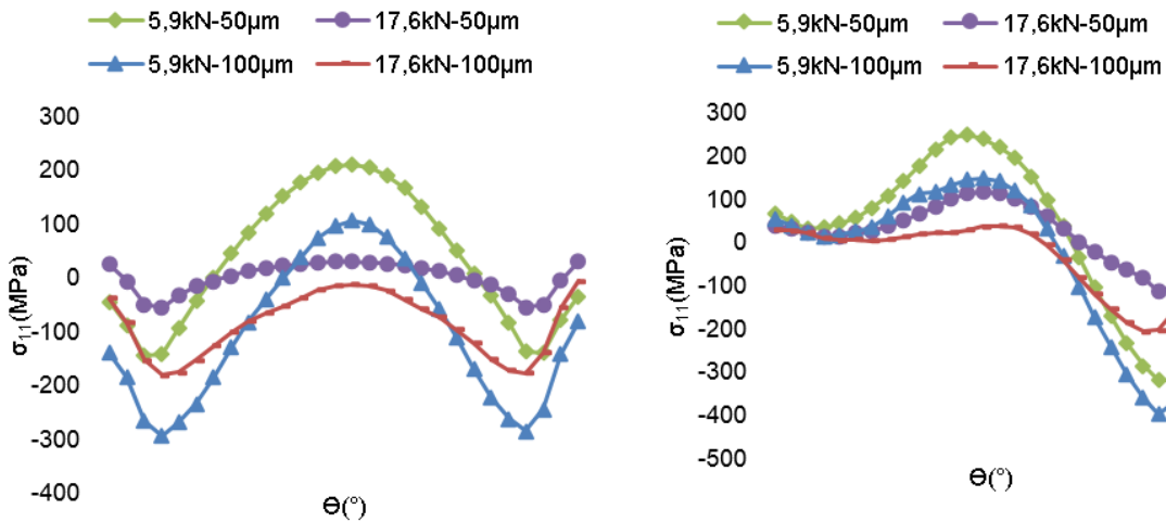
Figure A1. 8 : Evolution des contraintes \sigma_{11} suivant le chemin PC_i en fonction de la précontrainte et de l'interférence : phase de la précontrainte (à gauche) et du chargement extérieur (à droite)
