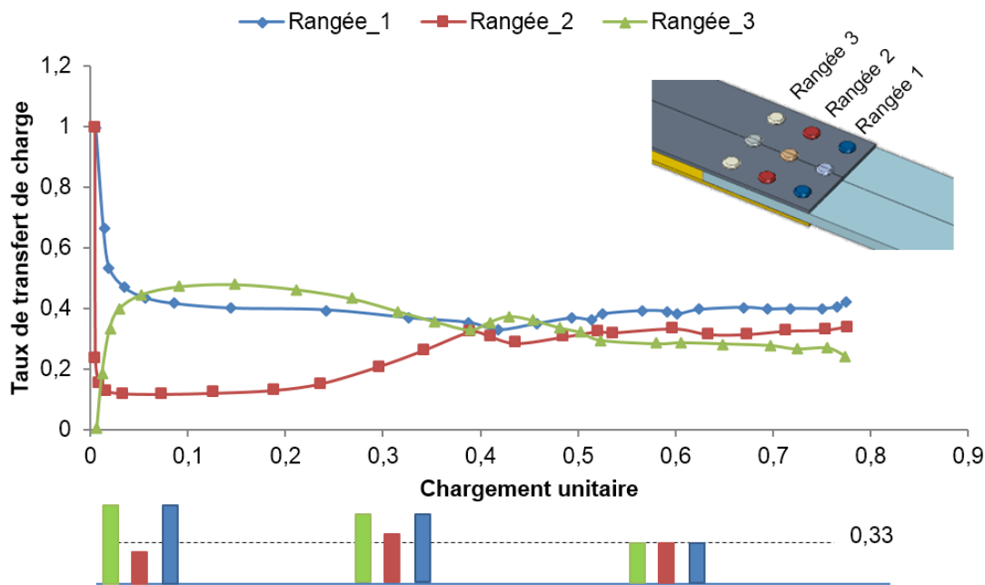
Figure 2. 25 : Taux de transfert de charge pour les 3 rangées d'assemblage à 9 fixations
