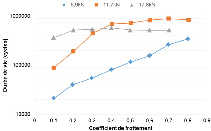
Figure 5.16 : Effet du coefficient de frottement à l'interface sur la durée de vie pour un chargement de 160MPa et pour différents niveaux de précontrainte
