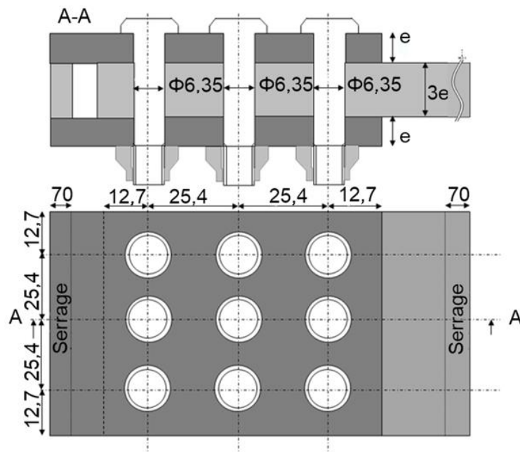
Figure 4. 16 : Assemblage à 9 fixations (dimensions en mm)
