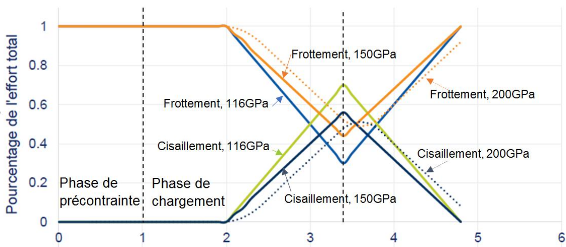
Figure 5.17 : Répartition de l'effort externe pour différents modules de Young de la fixation
