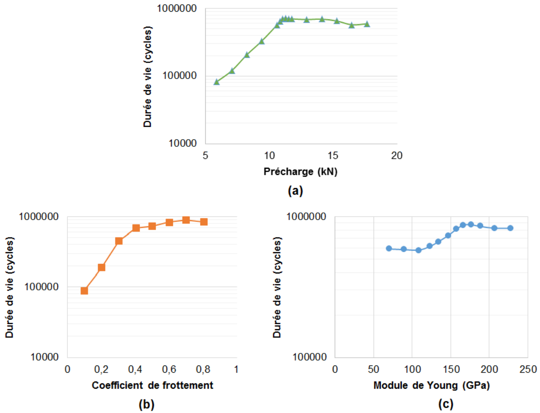
Figure 5. 15: Effet de la précontrainte (a), du coefficient de frottement à l'interface (b) et du module d'élasticité des fixations (c) sur la durée de vie de l'assemblage de référence pour un chargement de 160MPa
