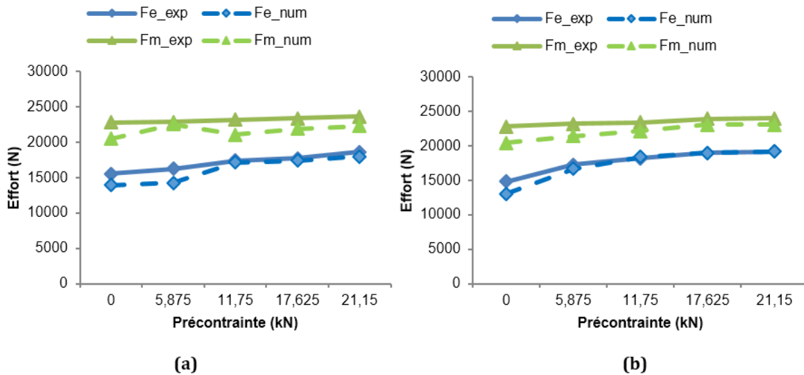
Figure 5. 6 : Comparaison entre le comportement statique numérique et expérimental pour un assemblage en simple cisaillement ajusté (a) et avec interférence de -50\mu\text{m} (b)
