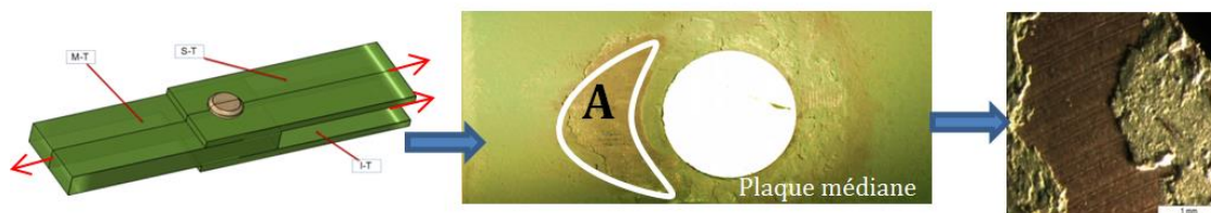
Figure 4. 10 : Observation de l'état de surface à l'interface
