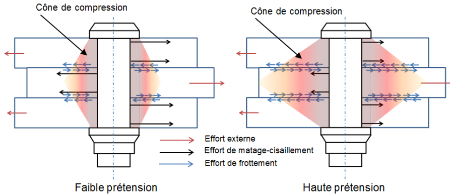
Figure 2. 10 : Schématisation des transferts d'efforts sous faible et haute précontrainte
