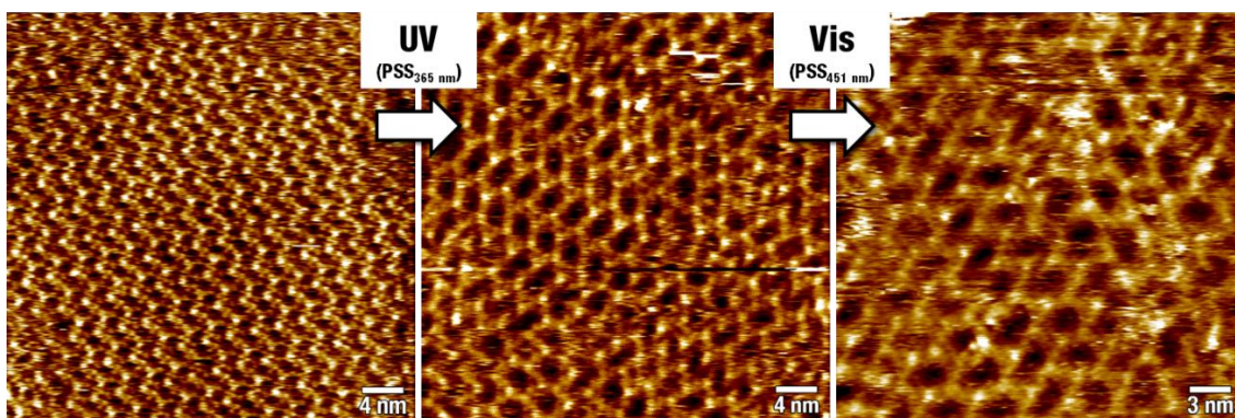
Figure 2. Images STM de 1 enregistrées à l'interface entre un substrat de graphite (HOPG) et une solution ( c = 10 \mu\text{M} ) de 1 en acide 1- heptanoïque. À gauche, pas de rayonnement lumineux. Centre, irradiation in-situ avec lumière UV à l'état photostationnaire (PSS, \lambda_{\text{max}} = 367 \text{ nm} ). À droite, irradiation ultérieure in-situ avec lumière visible (PSS, \lambda_{\text{max}} = 451 \text{ nm} ).
