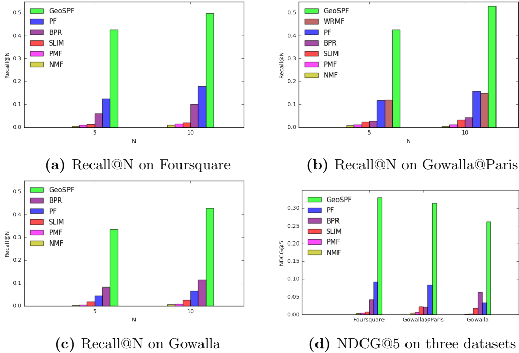
Figure A.4: Comparaison des performances avec des approches alternatives pour trois jeux de données : Foursquare, Gowalla@Paris et Gowalla. Nous traçons le Recall@N pour N = 5 et N = 10 sur les figures A.4a, A.4b et A.4c. Nous traçons le NDCG@5 sur la figure A.4d. Nous observons que GeoSPF dépasse de manière significative les autres modèles sur les trois jeux de données pour les trois mesures de qualité choisies.
