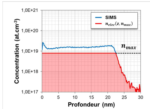
Figure III-4 : Graphe de la concentration en fonction de la profondeur pour les profils SIMS et n_{elec}(x, n_{max}) . La ligne en pointillés rouge illustre le niveau maximal de concentration n_{max} .
