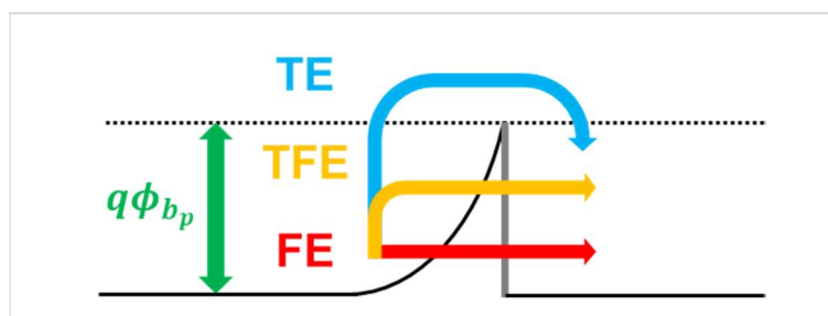
Figure V-1 : Représentation schématique des trois modes d'émission décrits par Crowell et Rideout : l'émission thermo-ionique (TE), par effet tunnel (FE) et thermo-électronique (TFE).
