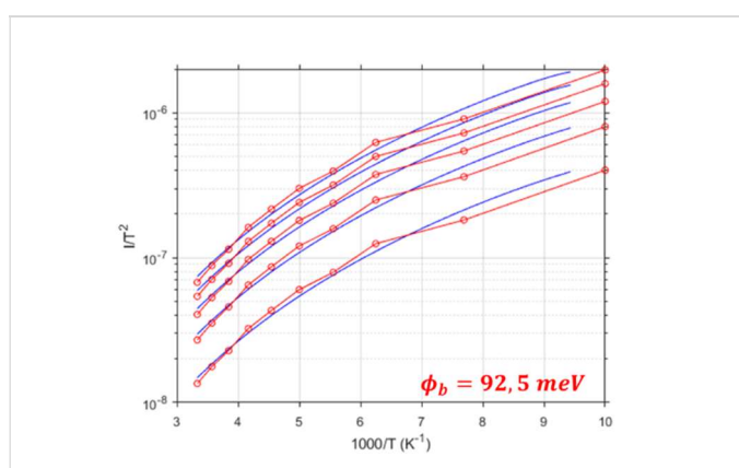
Figure V-27 : Courbes d'Arrhenius pour un contact PtSi/p-Si modulé par procédé IBS-BF 2 pour des températures entre 160K et 300K et des tensions de 0,2 V à 1 V. En rouge, les courbes expérimentales et en bleu les courbes simulées.
