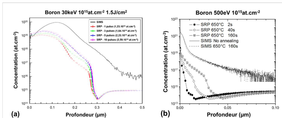
Figure IV-20 : (a) Profils de concentrations chimiques (SIMS) et actives (SRP) en fonction de la profondeur pour une couche de Si implantée bore (30keV à 10 15 at.cm -2 ) et activée par laser à une énergie de 1,5 J.cm -2 pour 1, 3, 5 ou 10 pulses successifs. (b) Profils SRP et SIMS d'une implantation de bore (0,5 keV à 10 15 at.cm -2 ) et activée par recuit RTA (spike/soak) à différents temps (2, 40 et 160 secondes).
