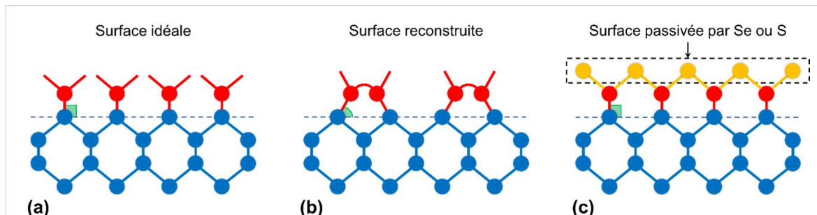
Figure I-28 : Représentation schématique d'un cristal de silicium observée selon la direction [110] pour une surface idéale (a), reconstruite (b) et passivée par une monocouche de Sélénium ou de Soufre (c) (figure inspirée de [TAO-03]).
