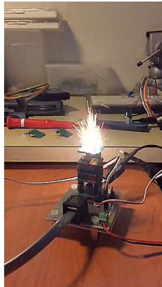
FIGURE 4.8 – Photo illustrant la mise à feu des micro-inflammateurs sur le module taille réelle
