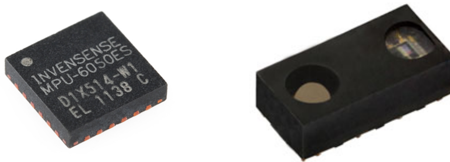
FIGURE 4.3 – Photo d'un accéléromètre (gauche) et d'un émetteur/récepteur IR (droite)
