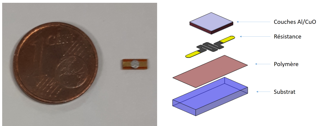
FIGURE 2.3 – Photo (gauche) et principe (droite) d'un micro-inflamateur - LAAS-CNRS
