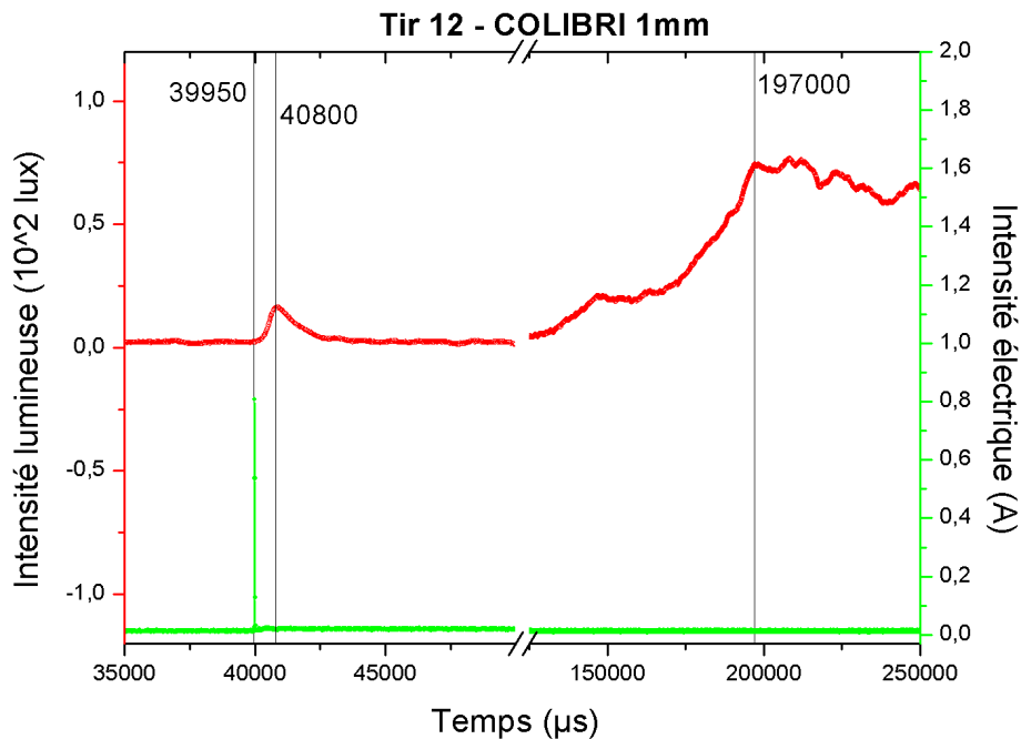
FIGURE 2.18 – Intensités lumineuses et électriques en fonction du temps pour un tir de micro-inflamateur à 1mm de 10mm 3 de COLIBRI
