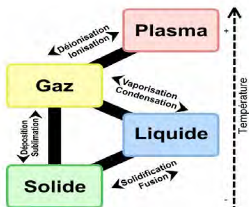
Figure 1 : Illustration des différents états de la matière
