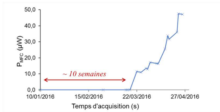
Fig. 1.16. Puissance générée par la BMFC #7 lors de son démarrage avec une résistance de 3 kΩ à ses bornes
