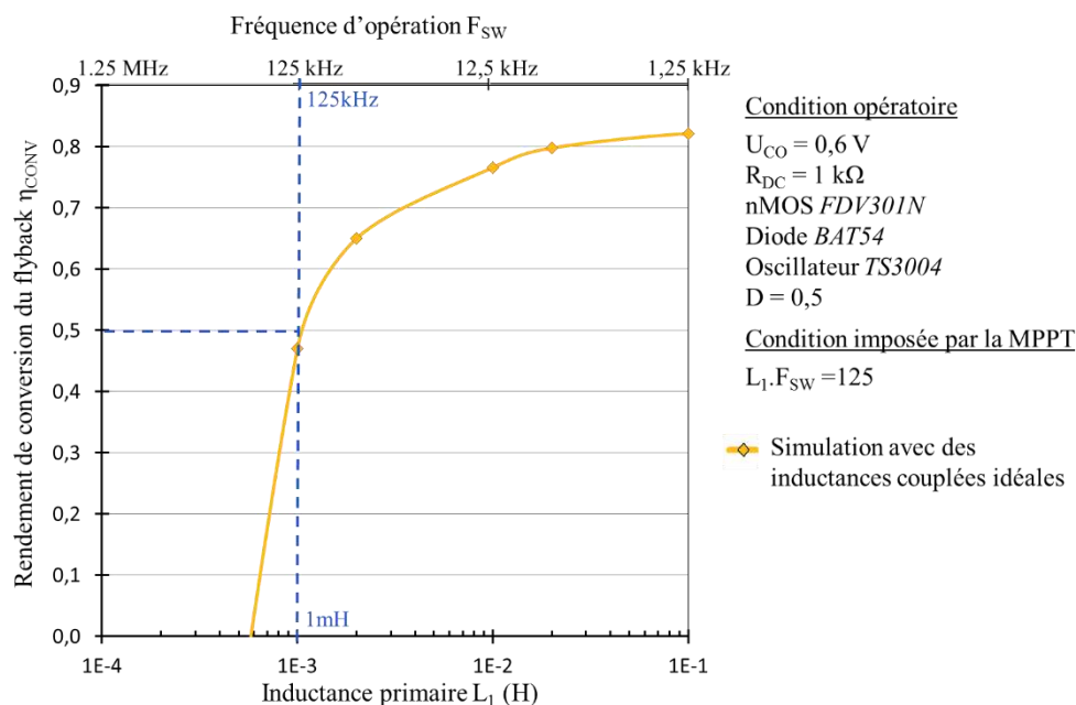
Fig. 4.3. Rendement de conversion du flyback \eta_{CONV} en fonction de l'inductance primaire L_1 lors d'un travail au MPP pour une puissance d'entrée de 90 \mu W .
