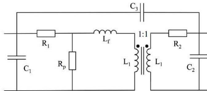
Fig. 3.13. Modèle électrique des inductances couplées.
