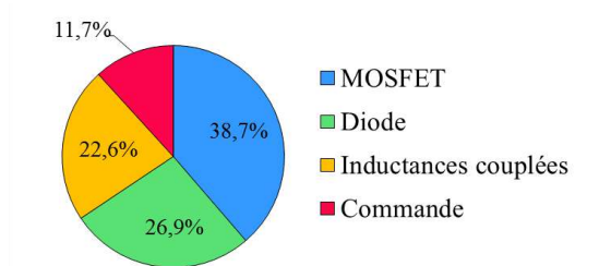
Fig. 4.14. Répartition des pertes au sein du flyback déterminée en simulation pour les inductances couplées #8.
