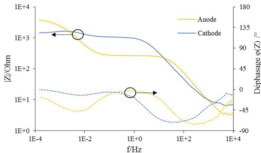
Fig. 2.14. Diagramme de Bode de l'anode et de la cathode d'une BMFC relativement à une électrode de référence ECS. Le module |Z| est en trait plein, le déphasage \varphi(Z) en pointillé.
