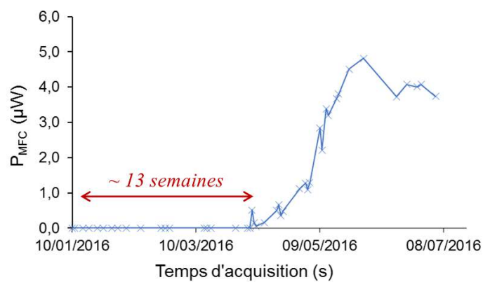
Fig. 1.17. Puissance générée par une BMFC conçue avec les sédiments du lac de l'Ovalie lors de son démarrage avec une résistance de 3 kΩ à ses bornes
