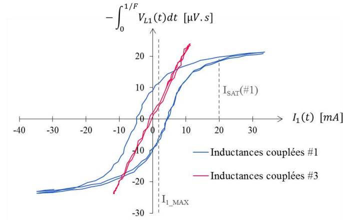
Fig. 4.5. Courbe statique d'aimantation des inductances couplées #1 et #3.
