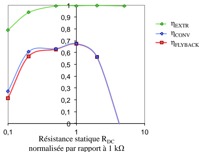
Fig. 5.17. Influence de la résistance statique R_{DC} sur les rendements du flyback utilisant le MPP-tracking (résultats expérimentaux).
