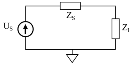
Fig. 3.2. Principe de l'adaptation d'impédance.
