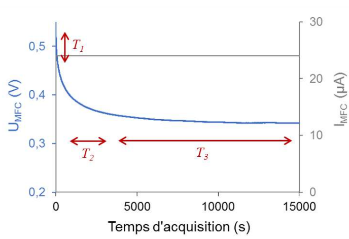
Fig. 1.21. Mise en évidence du régime transitoire de BMFC #8
