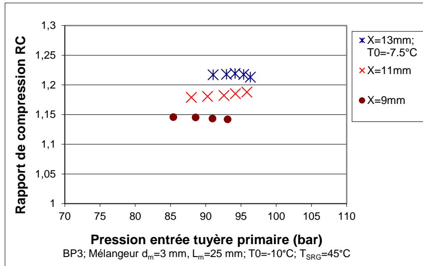
Figure 3.16 : Effet de la position de la tuyère primaire BP3 sur le rapport de compression en fonction de la pression à l'entrée de la tuyère primaire avec le mélangeur de diamètre 3 mm pour des températures d'évaporation et de sortie refroidisseur de gaz constantes
