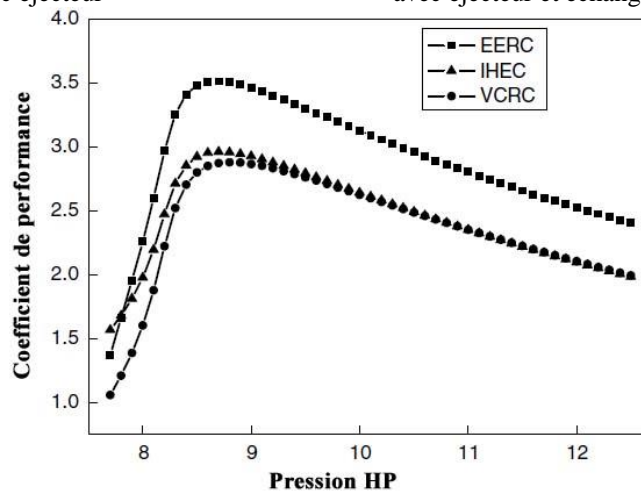
Figure 1.29 : Coefficient de performance du cycle équipé d'éjecteur, du cycle avec échangeur de chaleur et du cycle conventionnel en fonction de la pression HP étudié par Deng et al [50]
