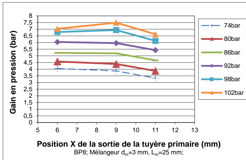
Figure 3.33: Gain en pression en fonction de la position de la tuyère primaire pour différentes pressions à l'entrée de la tuyère primaire BP8 avec le mélangeur de diamètre 3 mm
