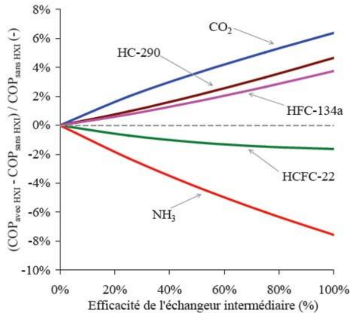
Figure 1.15 : COP relatif avec/sans échangeur de chaleur intermédiaire (0 °C / 35 °C)
