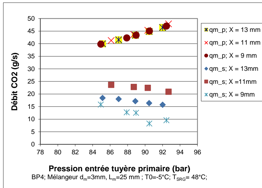
Figure 3.8 : Effet de la position de la tuyère primaire BP4 sur les débits primaire et secondaire pour différentes pressions à l'entrée de la tuyère primaire avec le mélangeur de diamètre 3 mm et pour des températures constantes
