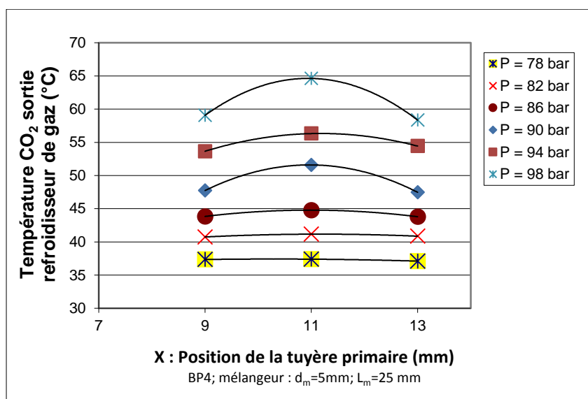
Figure 3.23 : Température CO 2 à la sortie du RGen en fonction de la position de la tuyère primaire BP4 avec le mélangeur de diamètre 5 mm pour diverses pressions à l'entrée de la tuyère
