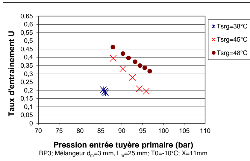
Figure 3.38 : Effet de la température à la sortie du refroidisseur de gaz sur le taux d'entraînement pour différentes pressions à l'entrée de la tuyère primaire BP3 avec le mélangeur de diamètre 3 mm
