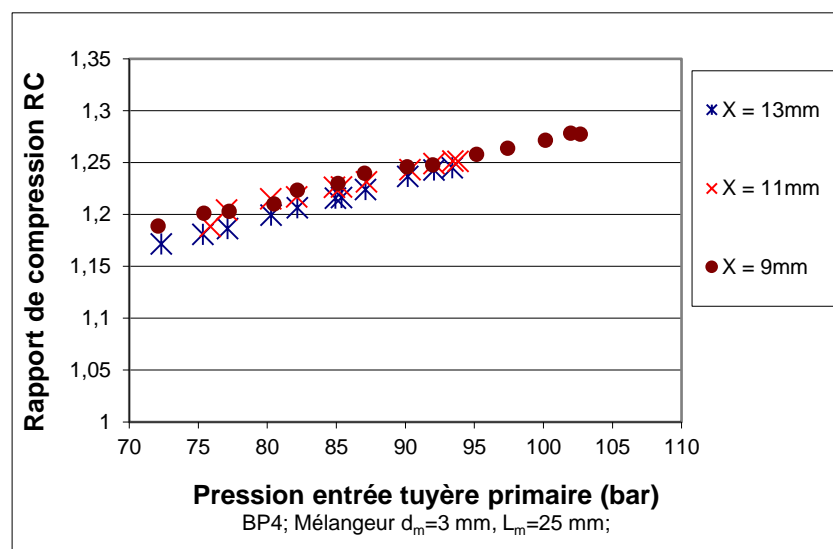
Figure 3.2 : Effet de la position de la tuyère primaire BP4 sur le rapport de compression pour différentes pressions à l'entrée de la tuyère avec le mélangeur de diamètre 3 mm
