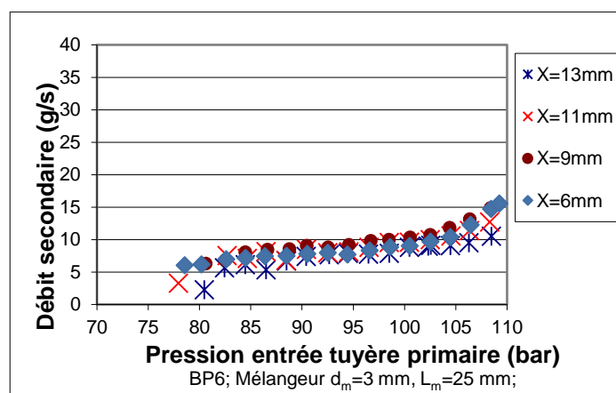
Figure 3.29 : Débit secondaire en fonction de la position X de la tuyère primaire pour différentes pressions à l'entrée de la tuyère primaire BP6 avec le mélangeur de diamètre 3 mm
