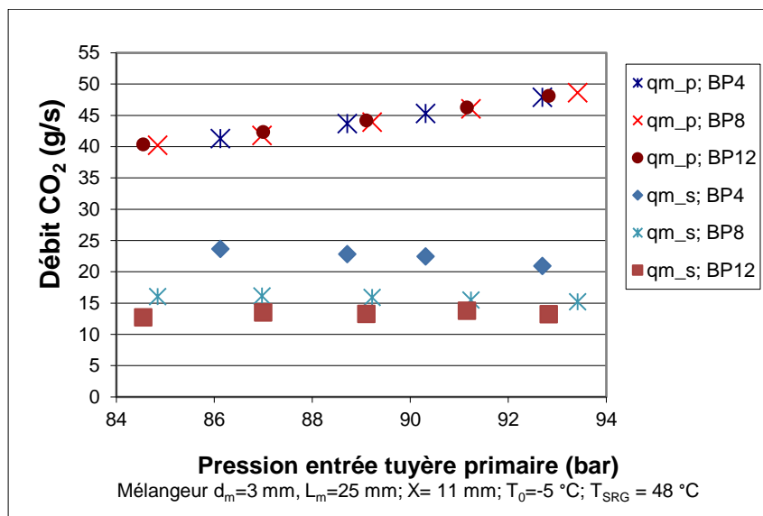
Figure 3.75 : Débits primaire et secondaire en fonction de la pression entrée tuyère primaire pour différents angles de divergent de la tuyère primaire (BP4 = 2° ; BP 8 = 5° ; BP 12= 7°) à températures constantes
