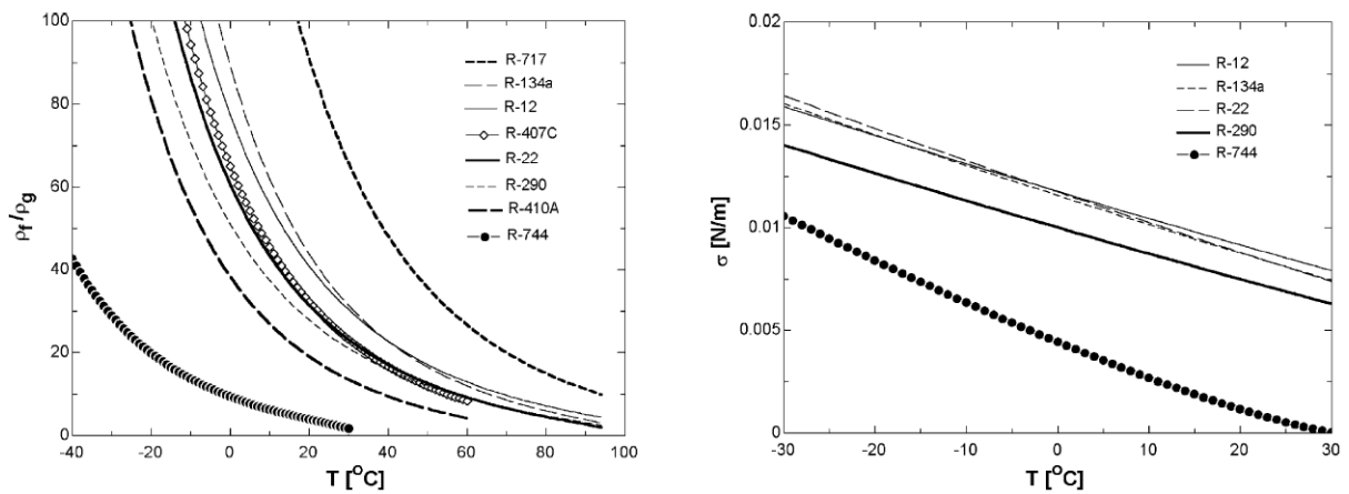
Figure 1.5 : \rho_{\text{liquide}}/\rho_{\text{gaz}} , et \sigma à saturation en fonction de la température
