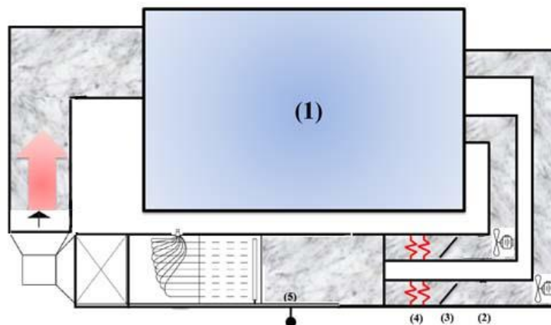
Figure 2.8 : Schéma du circuit d'air (source froide)
