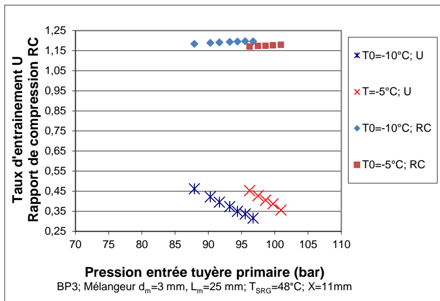
Figure 3.45: Rapport de compression et taux d'entraînement en fonction de la pression à l'entrée de la tuyère primaire BP3 avec le mélangeur de diamètre 3 mm pour diverses températures d'évaporation
