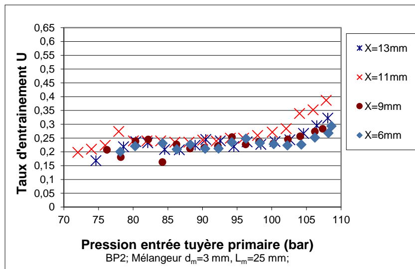
Figure 3.17 : Effet de la position de la tuyère primaire BP2 sur le taux d'entraînement pour différentes pressions à l'entrée de la tuyère primaire avec le mélangeur de diamètre 3 mm
