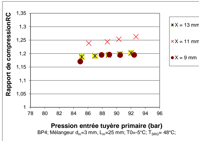
Figure 3.7 : Effet de la position de la tuyère primaire BP4 sur le rapport de compression RC pour différentes pressions à l'entrée de la tuyère primaire avec le mélangeur de diamètre 3 mm et pour des températures constantes
