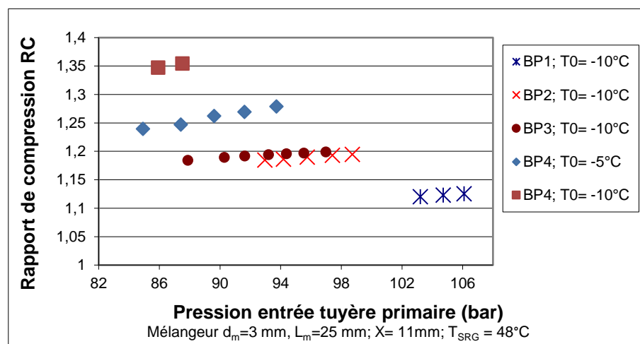
Figure 3.55 : Rapport de compression en fonction de la pression à l'entrée de la tuyère primaire avec le mélangeur de diamètre 3 mm et différents diamètres au col des tuyères primaires
