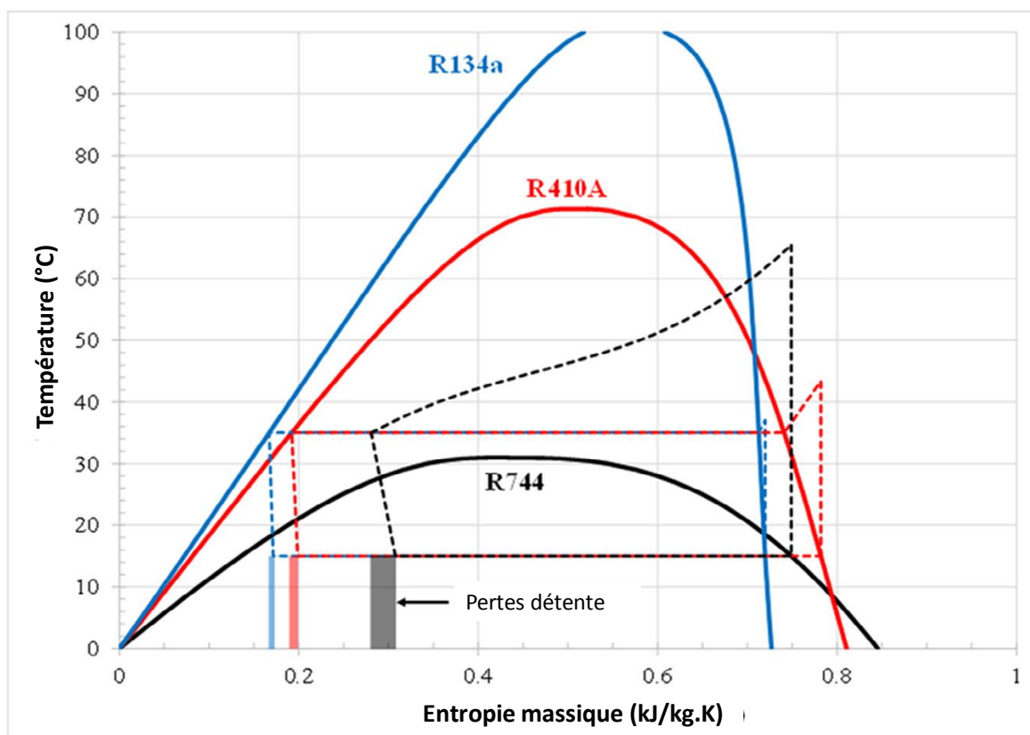
Figure 1.14 : Diagramme T-s du cycle à compression de vapeur avec détente isenthalpique pour le R744, le R410A et le R134a [108]
