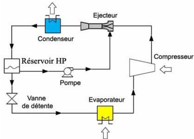
Figure 1.19 : Utilisation d'un éjecteur comme second étage de compression
