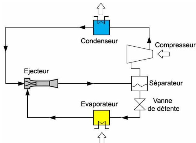
Figure 1.20 : Utilisation de l'éjecteur comme organe de détente
