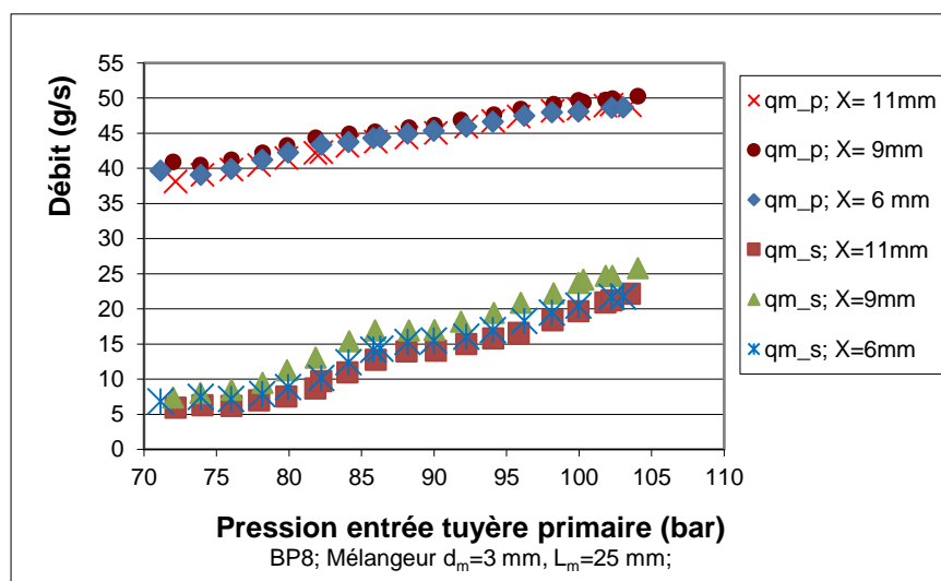
Figure 3.34 : Débits primaire ( q_{m_p} ) et secondaire ( q_{m_s} ) en fonction de la position de la tuyère primaire pour différentes pressions à l'entrée de la tuyère primaire BP8 avec le mélangeur de diamètre 3 mm
