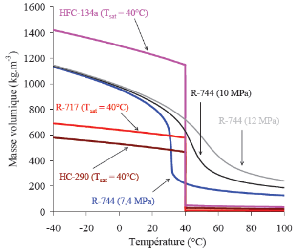
Figure 1.9 : Masse volumique de différents fluides frigorigènes en fonction de la température
