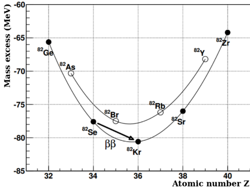
FIGURE 1.2 – Excès de masse en fonction du numéro atomique Z . Énergétiquement, une décroissance \beta simple est impossible pour le ^{82}\text{Se} . La \beta\beta vers le ^{82}\text{Kr} est alors permise.
