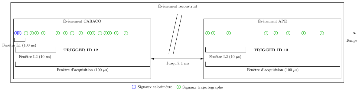
FIGURE 4.8 – Stratégie de construction d’un évènement prompt CARACO suivi d’un évènement retardé APE. La stratégie est équivalente pour le mode retardé DAVE.
