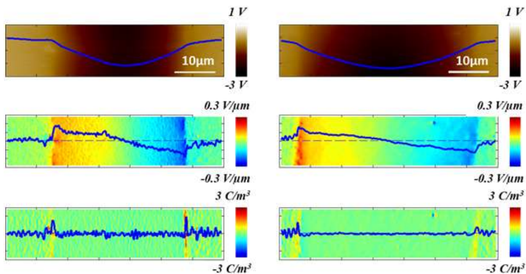
Figure 5 Comparaison du potentiel de surface (a; d), du champ électrique (b; e) et des cartes de densité de charge (c; f) pour un sandwich dont le LDPE a été traité en utilisant Al dans Laplace (rangée de gauche) et ABB (rangée de droite). La densité de charge est calculée en utilisant la méthode SG 2D.
