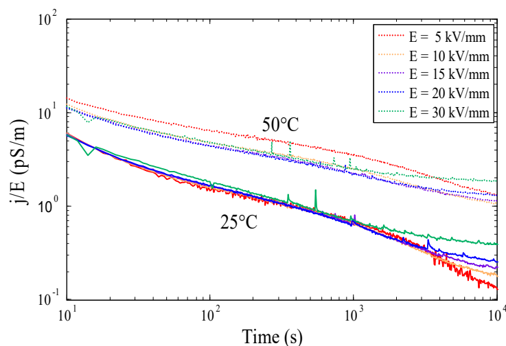
Figure 4 Transitoires de courant normalisés obtenus sur LDPE traité avec des couches de protection PI.
