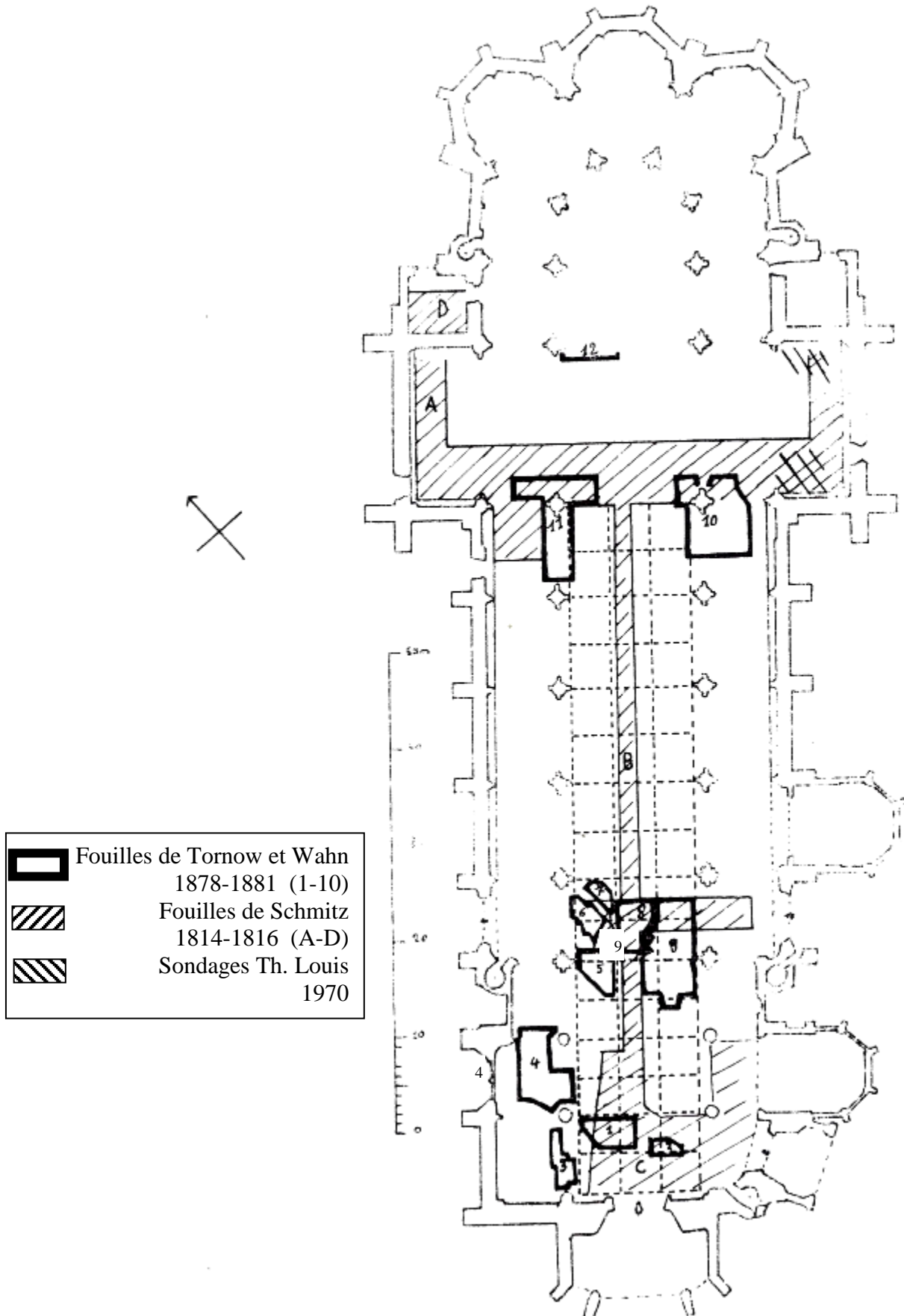
Fig. 11 - Chronologie des fouilles Plan établi par F. Héber-Suffrin, dans Églises de Metz dans le haut Moyen-Âge , 1982, pl. V.
