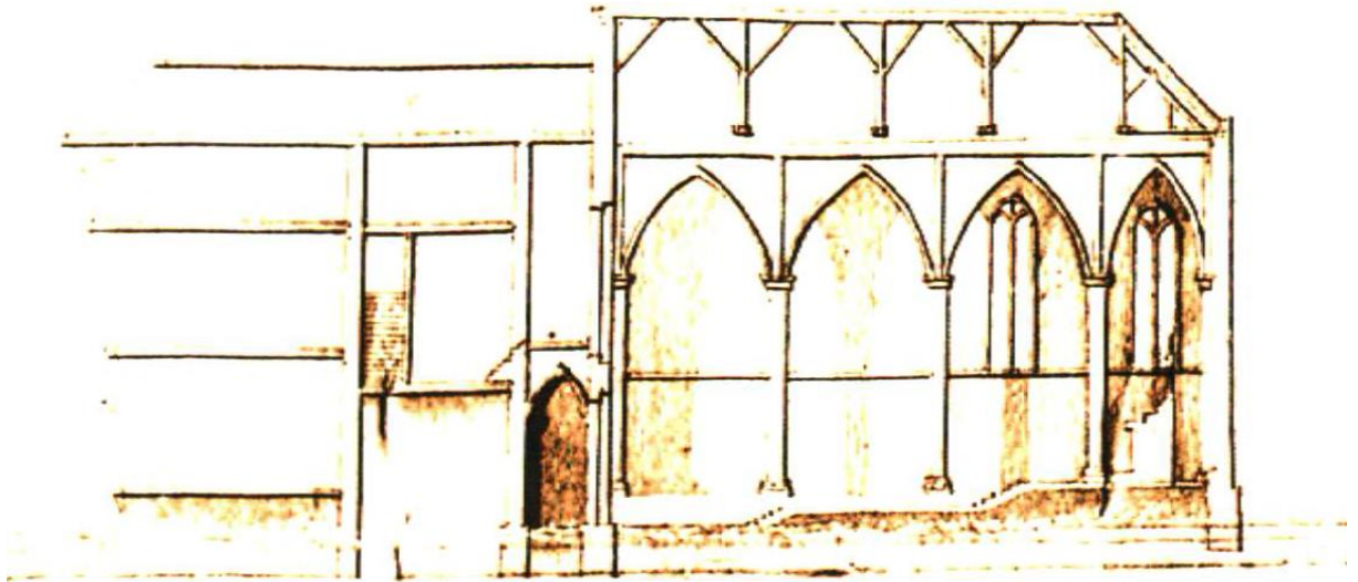
Fig. 7 - Coupe longitudinale sur la chapelle Saint-Pierre-le-Vieux. Détail du plan de la place d'Armes... J.A. Régner, 1754.
