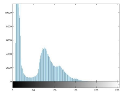
CHMF histogram
