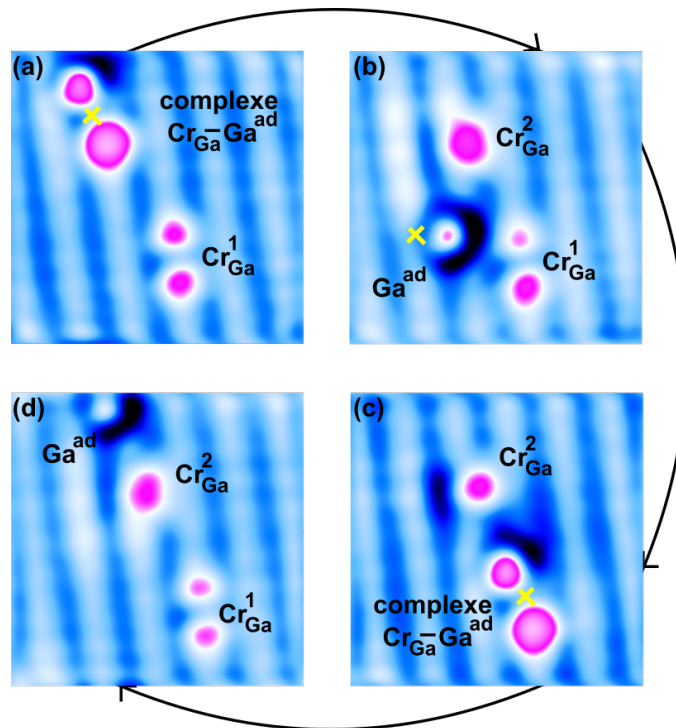
Fig. III.23: Images STM ( 3 \text{ nm} \times 3 \text{ nm} ; -1.5 \text{ V} ; 100 \text{ pA} ; 5 \text{ K} ) montrant la réversibilité du processus de création d'un \text{Cr}_{\text{Ga}}^1 (b) \rightarrow (c) \rightarrow (d) et l'irréversibilité du processus de création du \text{Cr}_{\text{Ga}}^2 (a) \rightarrow (b) \rightarrow (c) \rightarrow (d) à partir d'un complexe \text{Cr}_{\text{Ga}}-\text{Ga}^{\text{ad}} . Les croix jaunes indiquant l'emplacement de la pointe durant la variation de la tension de -1.5 \text{ V} à +1.7 \text{ V} sur les structures.
