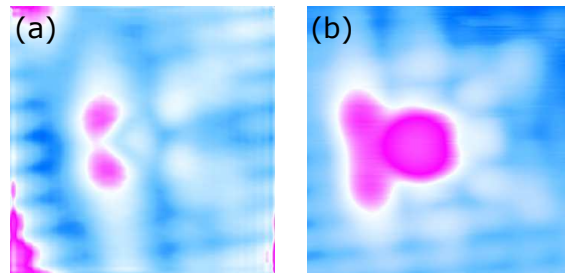
Fig. III.33: Images topographiques ( 3\text{ nm} \times 3\text{ nm} , 100\text{ pA} , 5\text{ K} ) d'un \text{Cr}_{\text{Ga}}^1 à V = +1.5\text{ V} (a) et d'un \text{Cr}_{\text{Ga}}^2 à V = +1.55\text{ V} (b).
