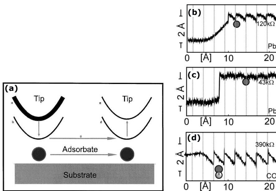
Fig. II.2: (a) Principe général de la manipulation latérale consistant à approcher la pointe au-dessus de l'adsorbate jusqu'à créer une interaction entre les deux ( \downarrow ) puis d'entraîner l'adsorbate dans le mouvement de la pointe jusqu'à un point cible ( \rightarrow ) et de couper leur interaction en éloignant la pointe à sa position d'imagerie ( \uparrow ). Selon les caractéristiques de la force pointe-adsorbate on distingue trois modes de manipulation latérale que l'on peut distinguer en visualisant la courbe de la variation de la hauteur de la pointe en fonction d'une ligne de scan sur un adsorbate : le mode de traction (b), le mode de coulissement (c) et le mode de répulsion (d) [106, 104].
