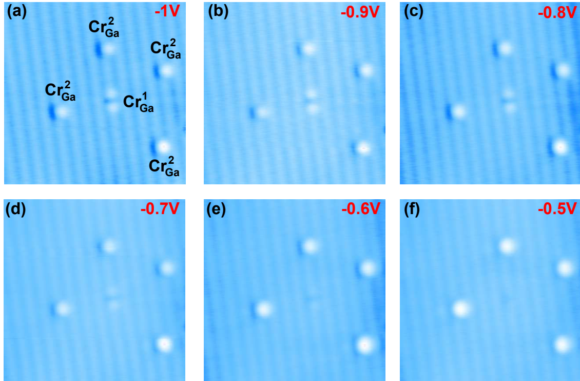
Fig. III.34: (a) \rightarrow (f) images STM (7 nm x 7 nm ; 100 pA ; 5 K) d'un \text{Cr}_{\text{Ga}}^1 et quatre \text{Cr}_{\text{Ga}}^2 à différentes valeurs de tensions négatives. Plus la tension tend vers les petites valeurs négative plus le contraste sur le \text{Cr}_{\text{Ga}}^2 augmente tandis qu'il diminue sur le \text{Cr}_{\text{Ga}}^1 jusqu'à disparaître à V = -0.5 \text{ V} .
