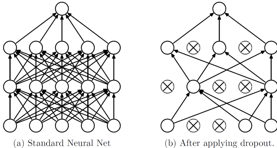
FIGURE 5.10 – Dropout : suppression de connexions entre les neurones entièrement connectés (source[8]).
