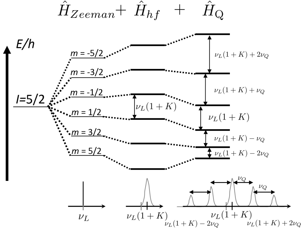
Figure 2: Spectre de RMN schématique pour I = 5/2 résultant de l'interaction Zeeman \hat{H}_{Zeeman} , de l'interaction hyperfine magnétique entre les noyaux et les électrons \hat{H}_{hf} qui entraîne le décalage de Knight K et de l'interaction quadrupolaire \hat{H}_Q donnant un pic central et des satellites internes et externes décalés de \pm\nu_Q et \pm 2\nu_Q , respectivement.
