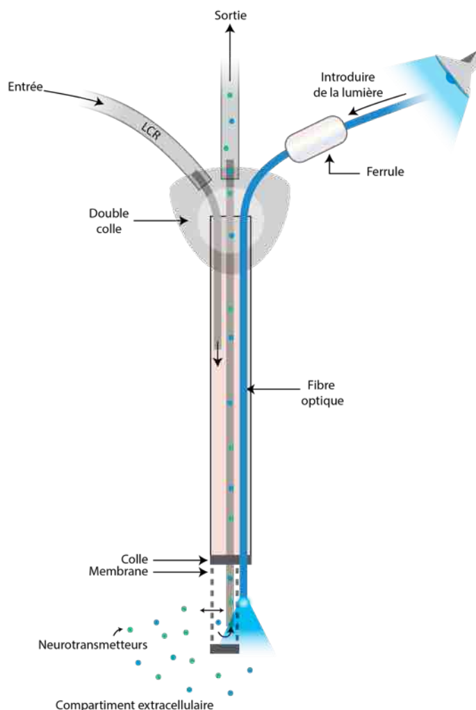
Figure 17. Composition une sonde microdialyse – optogénétique
