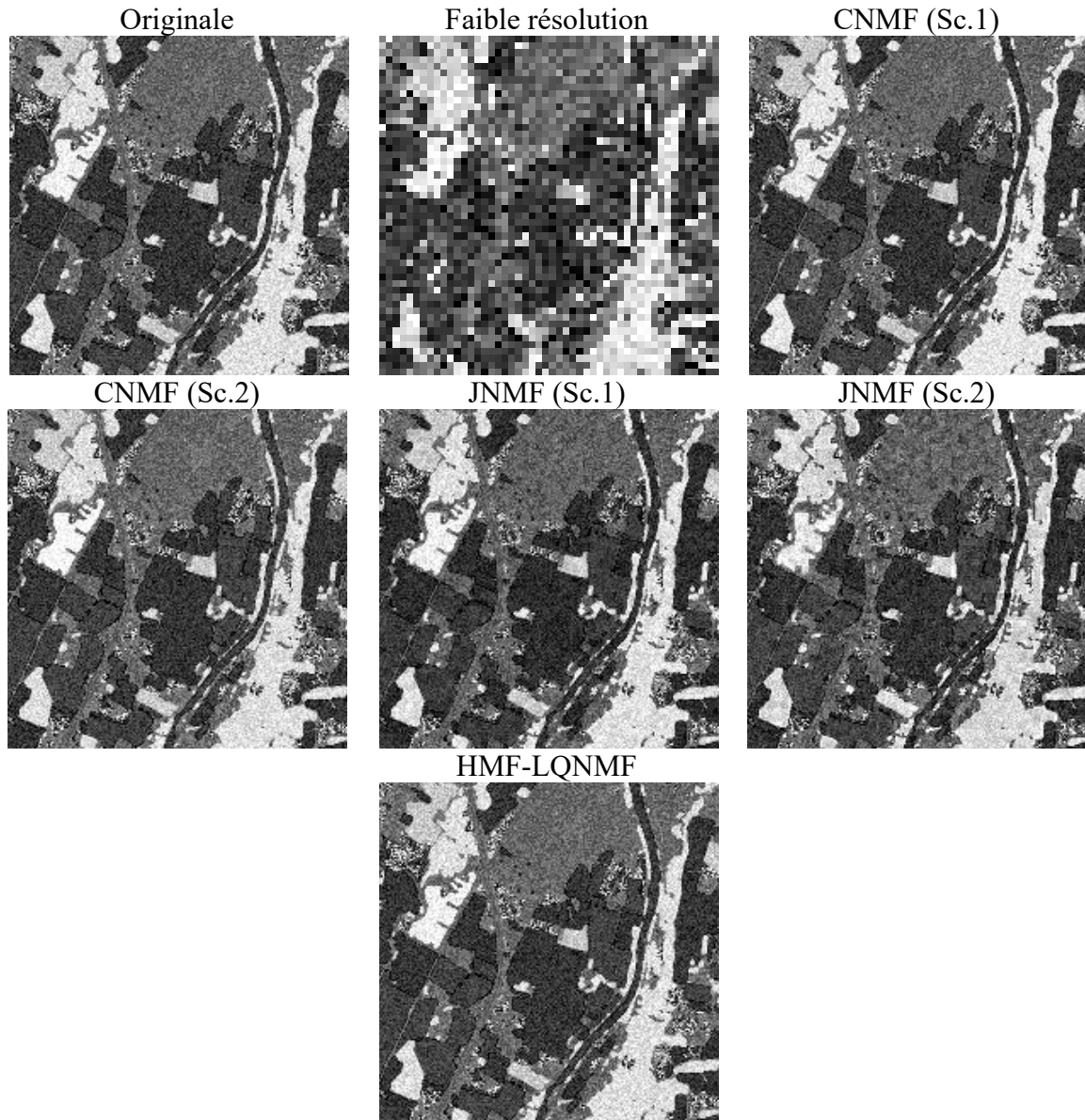
Figure 3.4 : Bande spectrale (dans la région de 0.815 \mu\text{m} ) de l'image hyperspectrale de référence (originale) à haute résolution spatiale, image hyperspectrale à faible résolution spatiale, images hyperspectrales à haute résolution spatiale fusionnée. - ensemble de données dataset 1.2, facteur d'échelle 4.
