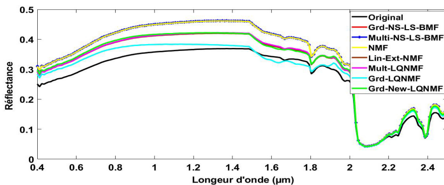
Figure 3.8 : Spectres originaux (spectres N°5-N°8) et spectres estimés - spectres de milieux urbains - données dataset 2.1 du Test 2- générées selon le modèle de mélange bilinéaire.
