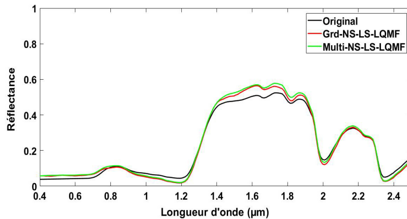
Figure 3.4 : Exemple d'un spectre original (dataset 1.2 du Test 1- générées selon le modèle de mélange linéaire-quadratique) avec ses estimées.
