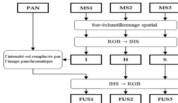
Figure 1.1 : Schéma de la méthode IHS [161].
