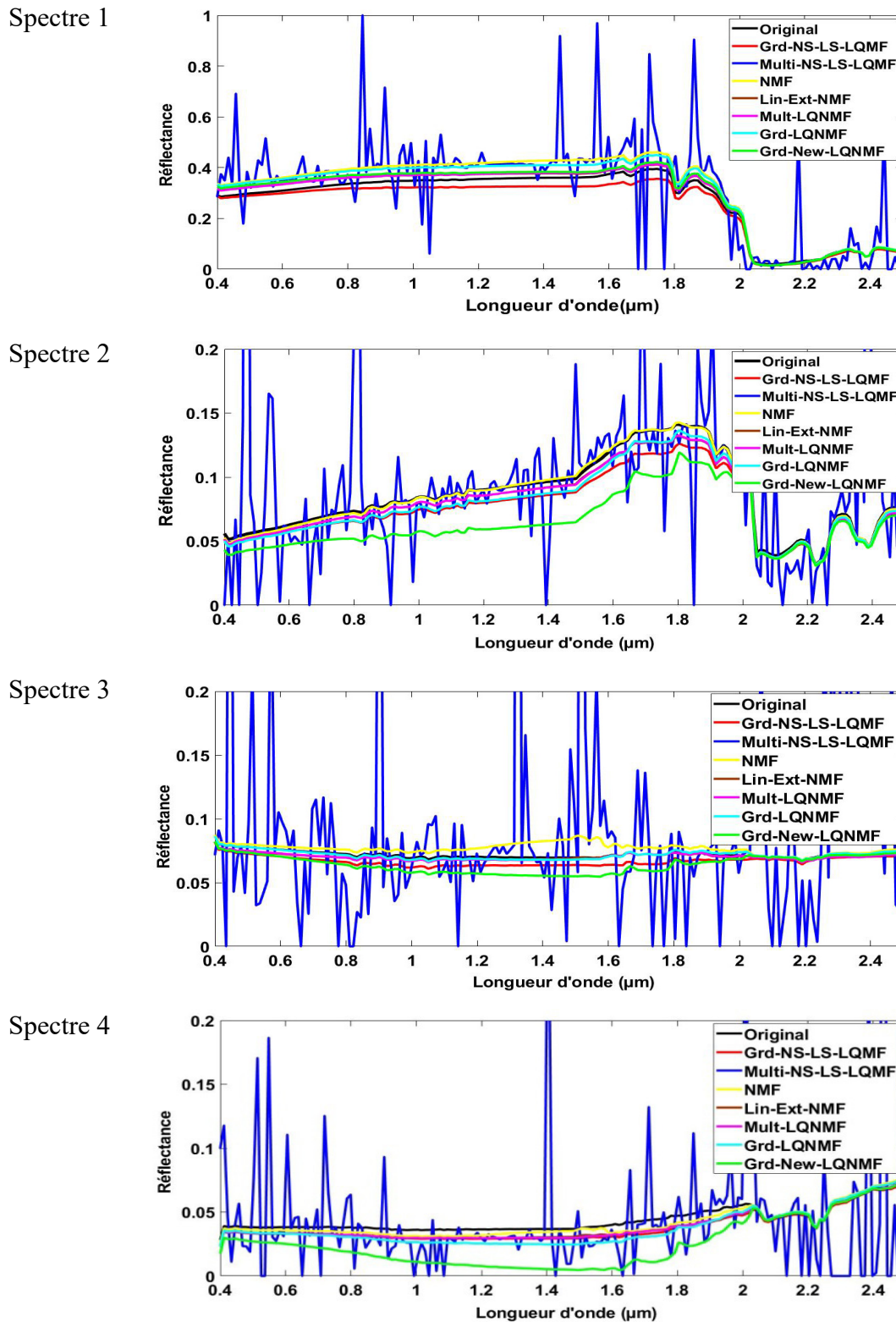
Figure 3.9 : Spectres originaux (spectres N°1-N°4) et spectres estimés - spectres de milieux urbains - données dataset 2.2 du Test 2- générées selon le modèle de mélange linéaire-quadratique.
