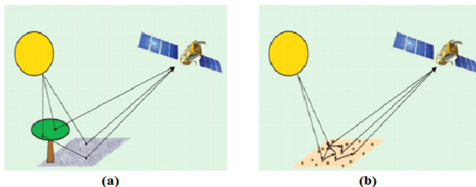
Figure 1.5 : Illustration du modèle de mélanges non-linéaires : (a) réflexions multiples, (b) mélange intime.
