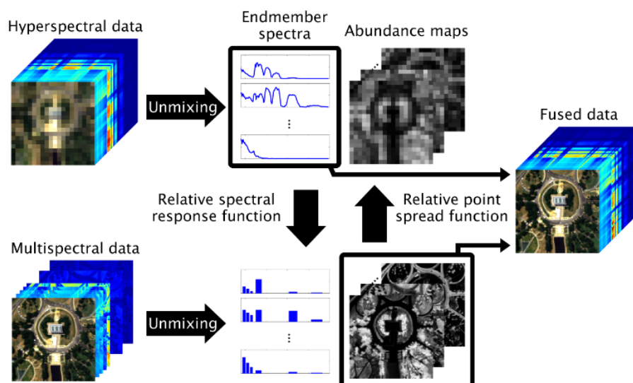
Figure 1.4 : Concept de la CNMF [156].
