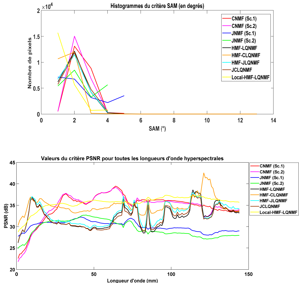
Figure 3.12 : Histogramme des valeurs du critère SAM (en degrés) et valeurs du critère PSNR (en décibels).
