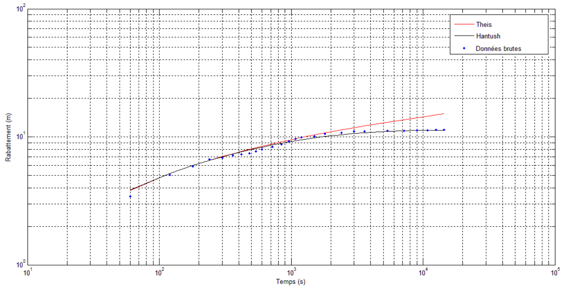
Figure 79 : Graphique du rabattement en fonction du temps suivant la comparaison Theis-Hantush pour le forage de Kamara
