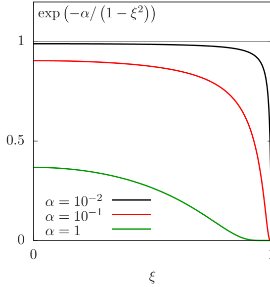
FIGURE 2.3 : Noyau C^\infty à support compact.
