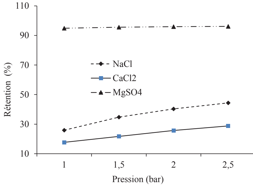
Figure 5.3 : Répartition de NaCl, CaCl 2 et MgSO 4 à 2 g/L en fonction de la pression sur NF270 ; P : 1 à 2,5 bars.
