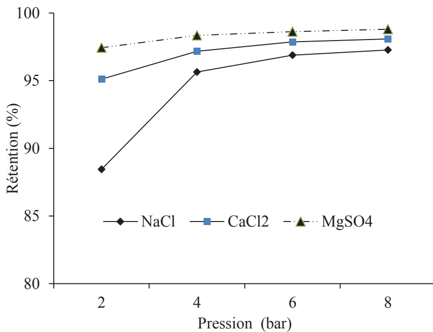
Figure 5.4 : Répartition de NaCl, CaCl 2 et MgSO 4 à 2 g/L en fonction de la pression sur TW30 ; P : 2 à 8 bars.
