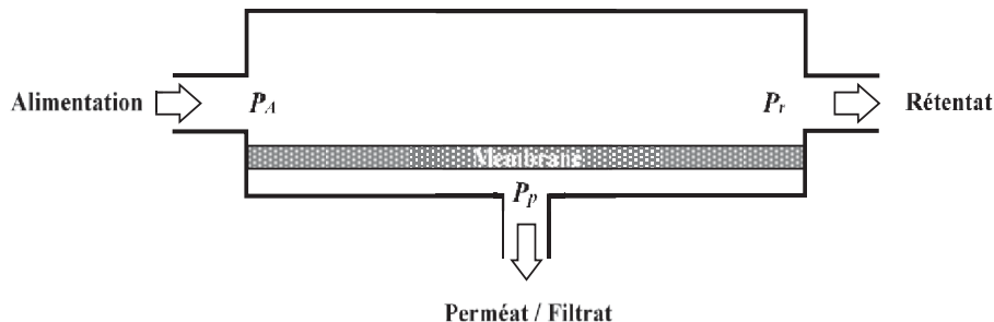
Figure 2.5 : Pression transmembranaire dans un module de filtration tangentielle.
