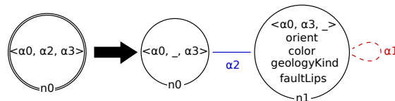
FIGURE 7.25 – Règle de duplication d'une arête
