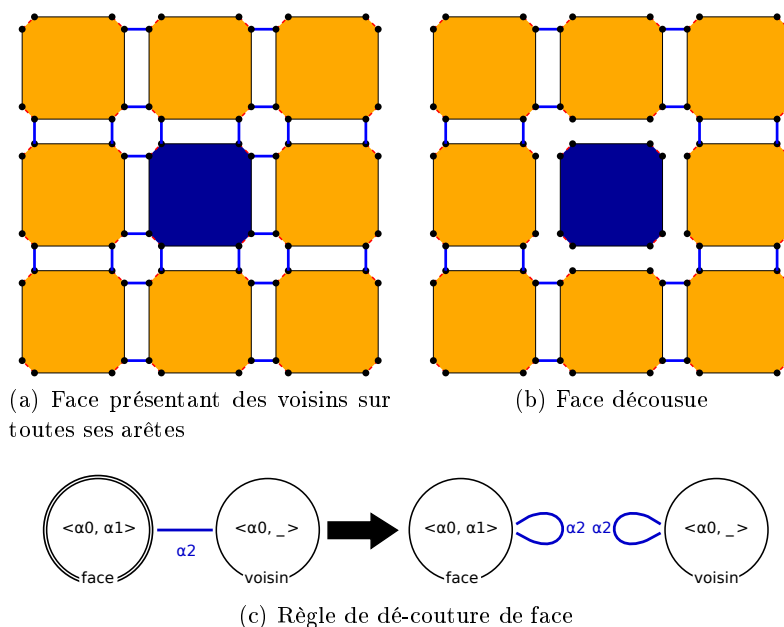
FIGURE 2.10 – Cas de dé-couture d'une face (ici bleue)
