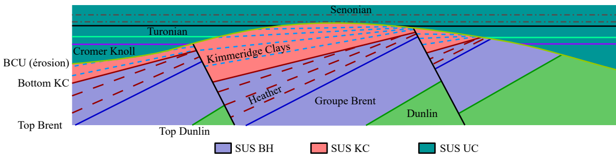
FIGURE 8.2 – Modèle ALWYN
