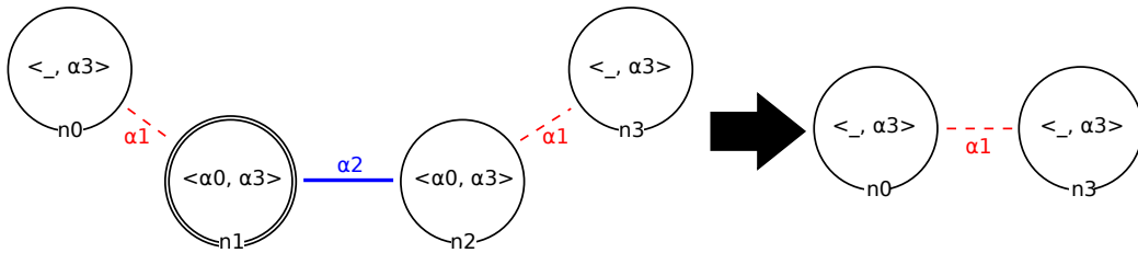
FIGURE 7.28 – Règle Jerboa permettant de fusionner 2 faces incidentes
