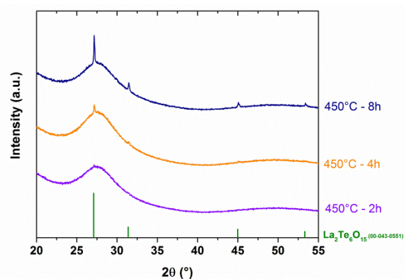
Figure II - 18 : Diffractogrammes des rayons X collectés sur les échantillons préfrittés obtenus par traitement thermique du verre à 450°C à différents temps de palier.
