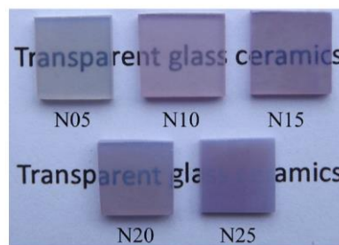
Figure III - 27 : Photographies de vitrocéramiques TBZ dopées \text{Nd}^{3+} (épaisseur : 2 mm) [35].
