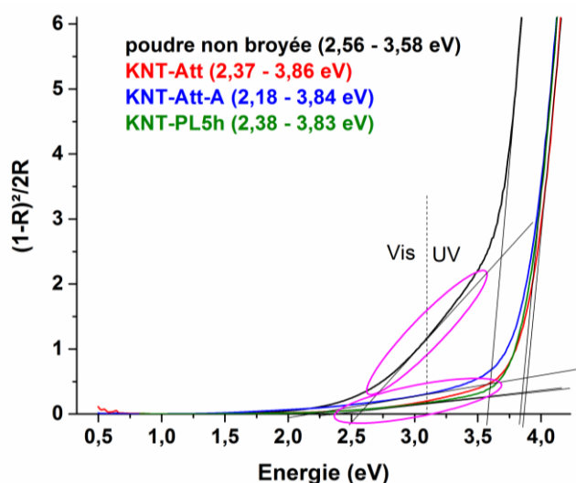
Figure IV - 69 : Détermination du gap optique par le modèle de Kubelka-Munk. Mise en évidence d'absorptions se produisant dans la gamme du visible (zones entourées).
