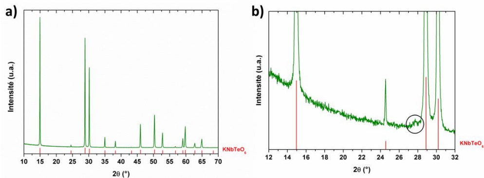
Figure IV - 44 : a) Diffractogramme enregistré sur la poudre dopée KNT1%HoAtt-A et b) zoom de la plage angulaire 12-32° en 2\theta . Diffractomètre Bruker D8 Advance – \text{CuK}\alpha_1 .
