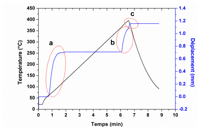
Figure II - 55 : Comportement type des essais SPS réalisés à T_{max} = 400^{\circ}C .
