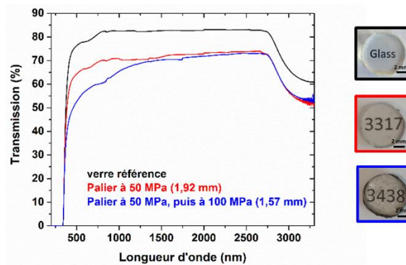
Figure II - 66 : Comparaison de la transmission de deux échantillons SPS (360°C - 0 min) dont le cycle de pression présente un palier (50 MPa) ou deux paliers (50, puis 100 MPa) en pression.
