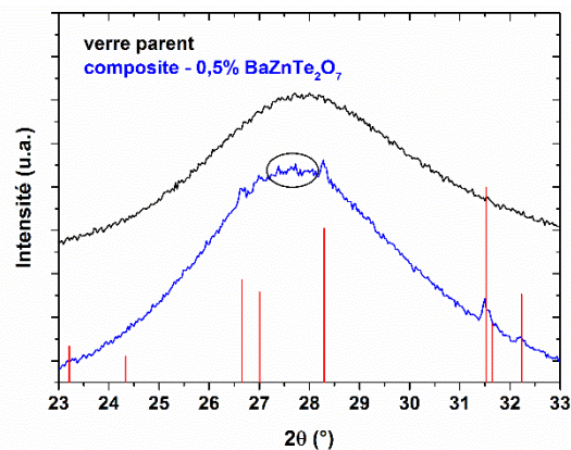
Figure II - 68 : Diagrammes de diffraction des rayons X enregistrés sur le verre de référence et pour un composite contenant 0,5wt.% en BaZnTe 2 O 7 .
