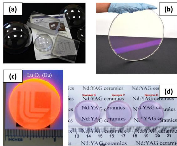
Figure I - 53 : (a) Lentilles et dômes (oxynitride d'aluminium AlON) [133], (b) (spinnelle MgAl 2 O 4 ) pour des armures transparentes [134], (c) scintillateurs (Lu 2 O 3 dopé Eu 3+ ) [135] et (d) céramique laser (YAG dopé Nd 3+ ) [136].
