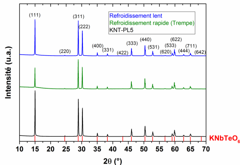
Figure IV - 60 : Diffractogrammes collectés sur la poudre KNT-PL5h, et sur cette même poudre ayant été traitée de nouveau à 750°C pendant 1h sous air, puis ayant subi un refroidissement lent ou un refroidissement rapide.
