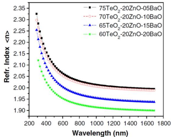
Figure II - 47 : Valeurs d'indices de réfraction en fonction de la longueur d'onde pour différents verres du système \text{TeO}_2\text{-ZnO-BaO} [49].
