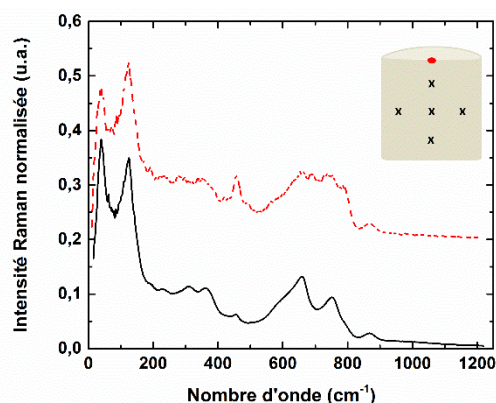
Figure III - 34 : Moyenne des spectres Raman enregistrés en différents points d'un échantillon traité thermiquement à 510°C pendant 5 min.
