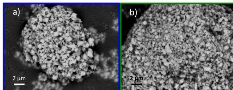
Figure IV - 45 : Micrographies MEB de la poudre dopée à 1% massique en \text{Ho}^{3+} avant (a) et après (b) post-traitement thermique à 400^\circ\text{C} .
