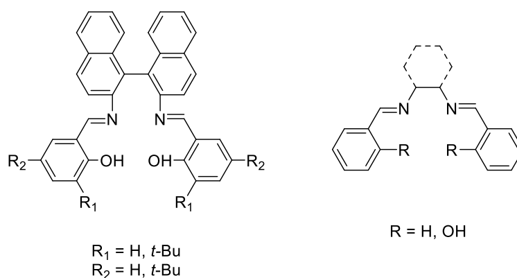
Figure 1.28 : Bases de Schiff utilisées pour le couplage entre le \text{CO}_2 et des époxydes
