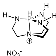
Figure 1.47 : Azaphosphatrane utilisé pour les additions de Michael et la réaction de Streker.
