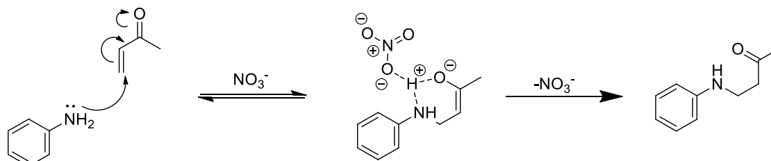
Figure 1.48 : Mécanisme de la réaction de Mickael et illustration de la "navette à proton"
