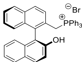
Figure 4.2 : Sel de phosphonium chiral utilisé pour la résolution cinétique d'époxyde 109
