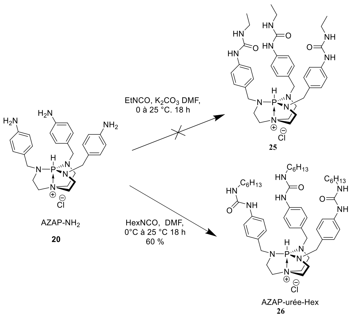
Figure 3.11 : Synthèse d'azaphosphatranes urée.
