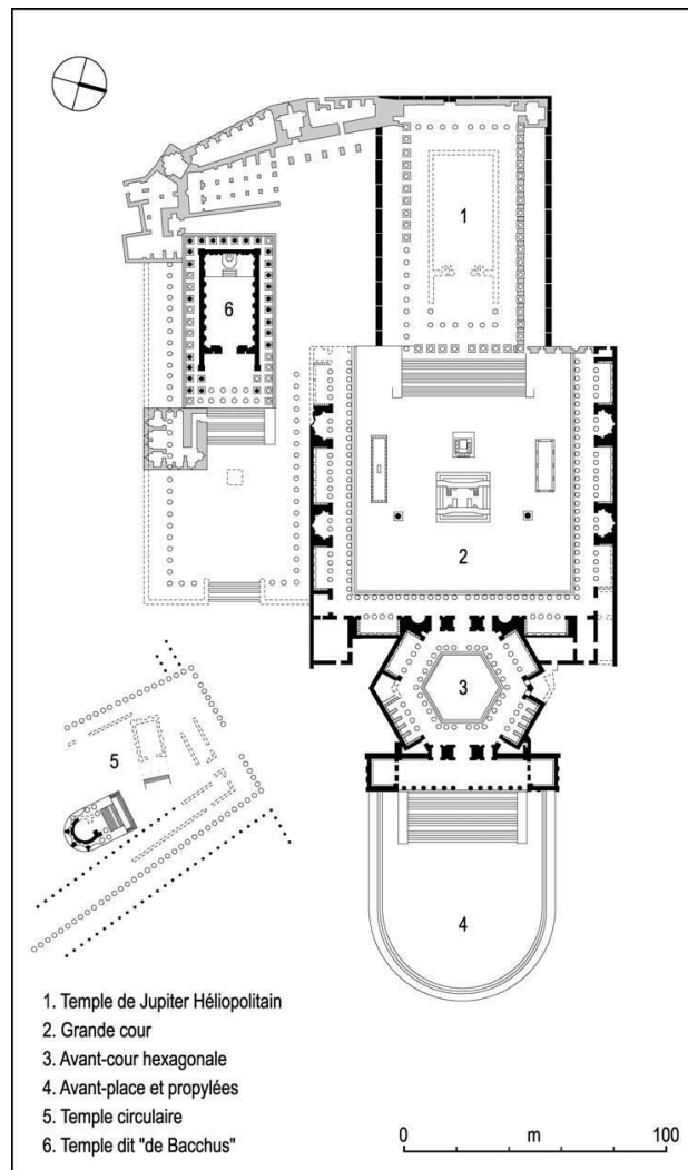
2- Plan du sanctuaire de Baalbek. D'après BRU (H.), 2011, p. 387, fig. 12.
