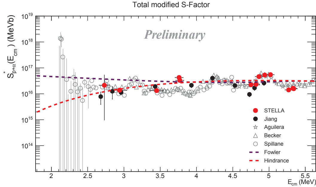
FIGURE IV.10 – Facteur astrophysique modifié sommé sur les voies proton et alpha obtenu avec STELLA (points rouges). Comparaison avec les données issues des Réfs. [13, 18–20] et les modèles de Fowler [21] et de suppression de la fusion [20]. Seules les incertitudes statistiques sont montrées pour nos résultats, et les barres horizontales représentent l'épaisseur de la cible, et non une erreur, la mesure étant placée à la position correspondante à l'énergie du faisceau au centre de cette dernière.
