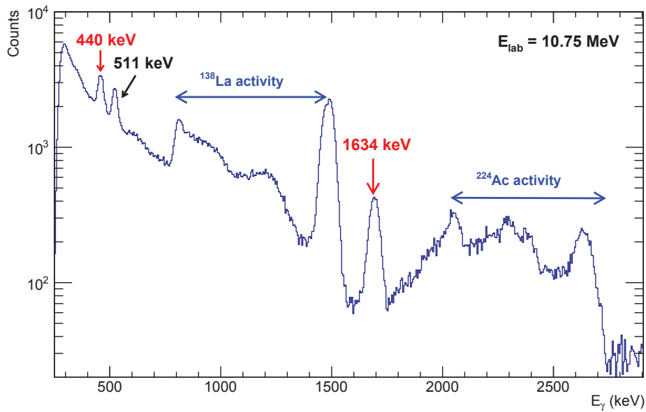
FIGURE III.4 – Spectre \gamma d'un \text{LaBr}_3(\text{Ce}) obtenu à E_{\text{lab}} = 10.75 \text{ MeV} . Les deux pics principaux provenant de la fusion ^{12}\text{C} + ^{12}\text{C} à E_{\gamma} = 440 \text{ keV} et E_{\gamma} = 1634 \text{ keV} sont indiqués en rouges sur la figure, tandis que la contribution de l'activité intrinsèque est indiquée en bleu.
