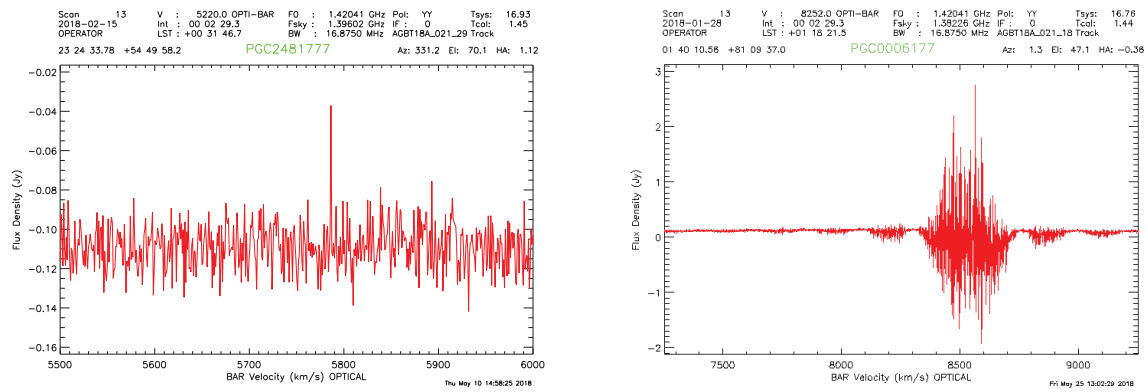
FIGURE 3.20 – Les deux types principaux d’interférences radio au GBT : à gauche une pic fin ( spike ), et à droite une émission large d’un radar ou d’un GPS.
