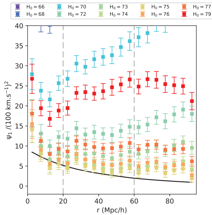
FIGURE 5.11 – Statistique \psi_1 en fonction de la distance de séparation r . La courbe noire correspond au modèle \Lambda\text{CDM} . L'estimateur \psi_1 a été calculé à partir des vitesses particulières des groupes CF3 pour différentes valeurs de H_0 : 66, 68, 70, 72, 73, 74, 75, 76, 77 et 79 \text{km/s/Mpc} .
