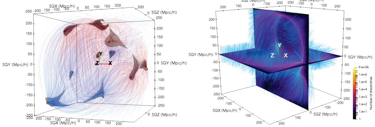
FIGURE 4.8 – Gauche : visualisation tri-dimensionnelle du champ de vitesse synthétique (lignes de flux rouges : point de vue avant ; lignes de flux bleues : point de vue arrière ). Les sphères rouges et bleues sont positionnées aux coordonnées des attracteurs et repousseurs respectivement. Les isosurfaces grises représentent des surdensités dans la matrice S telles que S > 700 (points de vues avant et arrière superposés). Droite : plans SGX-SGY et SGX-SGZ de l’histogramme des lignes de flux S (point de vue avant ), centrés respectivement en SGZ = 0 Mpc/h et SGY = 0 Mpc/h. L’échelle des couleurs est logarithmique afin de faciliter la visualisation. Les lignes de flux (point de vue avant ) sont représentées en bleu dans deux tranches d’épaisseur 50 Mpc/h centrées sur les deux plans.
