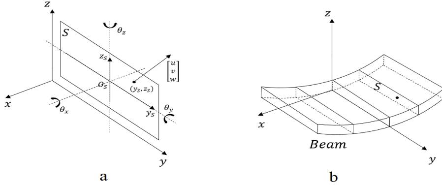
Figure 4.3: Cinématique
