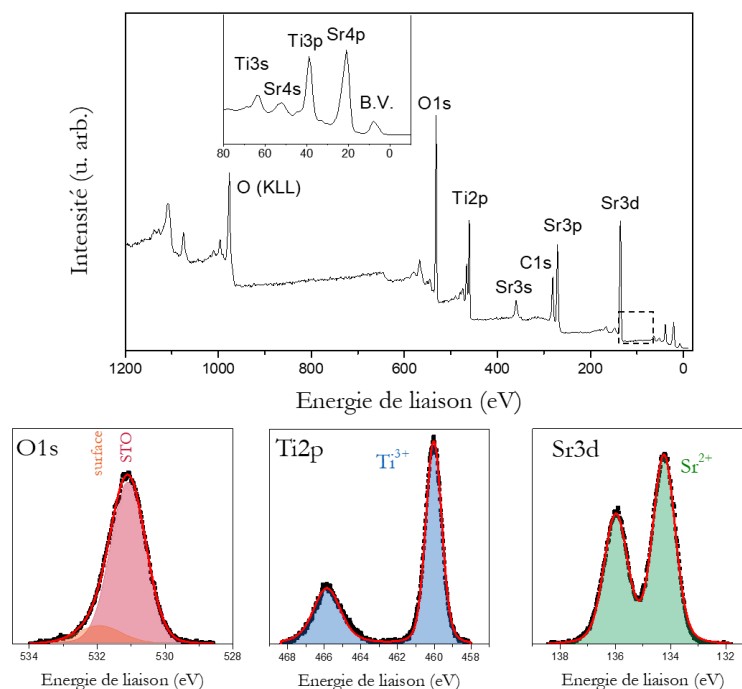
Figure 5.23 – Spectre global et niveaux de cœur O1s, Ti2p et Sr3d d'un substrat de STO pour une source AlK\alpha monochromatisée.
