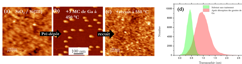
Figure 2.10 – Images AFM (a) d'un substrat de Si(111) recouvert de silice et (b) d'un dépôt de 3 MC de Ga à 450 °C sur ce substrat, (c) d'un dépôt de 3 MC de Ga à 450 °C suivi d'un recuit à 550 °C; (d) topographie de la surface du substrat SiO 2 /Si(111) (en vert) et de l'échantillon après recuit (en rouge).
