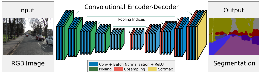
Fig. 4.13.: Schémas du réseau SegNet [Bad+15] développé par Badrinarayanan et al. L'architecture de ce réseau est très proche de celle de Noh et al. illustrée dans la figure 4.11 mais ne possède pas de partie entièrement connectée. Image tirée du papier [Bad+15].
