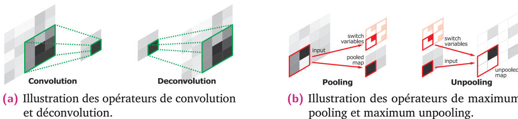
Fig. 4.12.: Opérateurs de convolution et de maximum pooling ainsi que leurs équivalents permettant la reconstruction des cartes de caractéristiques. Image tirée du papier [Noh+15].
