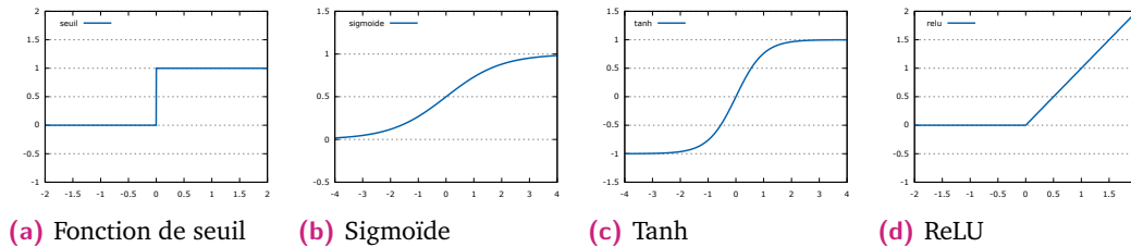
Fig. 2.2.: Les fonctions d'activations les plus connues. De gauche à droite : la fonction de seuil (historique mais inutilisable dans les réseaux d'aujourd'hui), Sigmoïde, Tanh et ReLU (Rectified Linear Unit).
