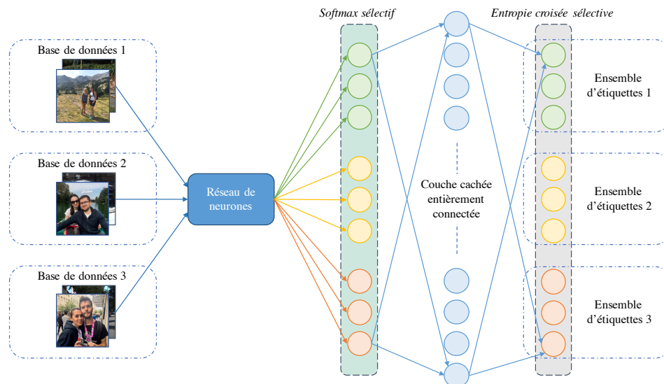
Fig. 5.3.: "Apprentissage joint avec partage de contexte" (AJPC). On ajoute une couche entièrement connectée (FC) après la sortie d'un premier réseau, pré-entraîné avec la stratégie d'apprentissage joint (figure 5.2). Une deuxième phase d'apprentissage est ensuite réalisée afin de prendre en compte les corrélations entre les classes sémantiques des différents ensembles d'étiquettes.
