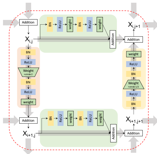
Fig. 6.3: Schéma détaillé des blocs composant notre GridNet. Les unités vertes sont résiduelles et gardes les dimensions des cartes de caractéristiques constantes entre l'entrée et la sortie. Les unités rouges sont convolutives. La partie "weight" en forme de losange est une couche convolutive avec un pas de deux, réduisant ainsi la résolution des cartes de caractéristiques et doublant leurs nombres. Les unités jaunes sont déconvolutives et doublent la résolution des cartes de caractéristiques avec une convolution stridée d'un pas d'un demi. BN = normalisation par batch.
