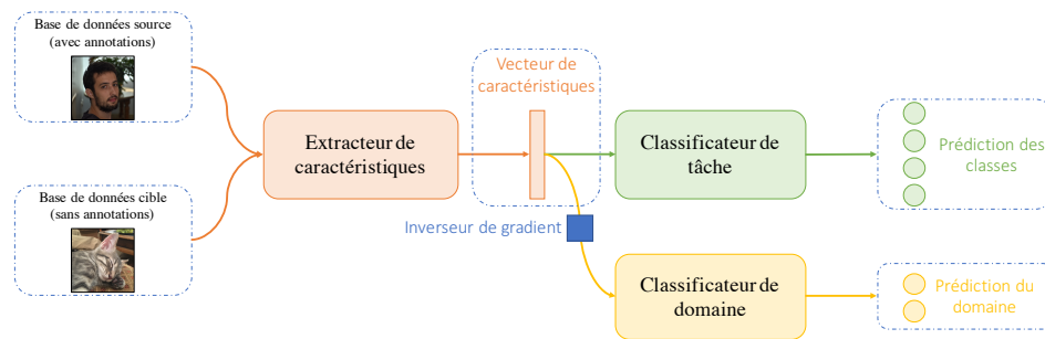
Fig. 5.4.: Illustration de l'inverseur de gradient de Ganin et Lempitsky [GL15]. L'extracteur de caractéristiques (en orange) extrait des caractéristiques utilisées par les deux classificateurs. Le classificateur de tâche (en vert) est entraîné à prédire les classes des images venant de la base de données source. Le classificateur de domaine (en jaune) est entraîné à prédire la provenance des images (base de données source ou base de données cible). L'inverseur de gradient (en bleu) inverse le gradient qui remonte du classificateur de domaine ayant pour effet d'entraîner l'extracteur de caractéristiques à extraire des données invariantes aux bases de données source et cible.
