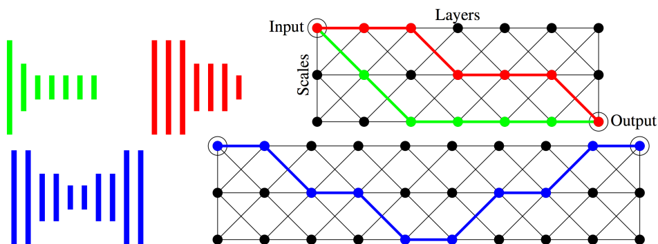
Fig. 6.1.: Schémas des Neural Fabrics de Saxena et al. [SV16]. Leurs structures sont très similaires à notre GridNet et permettent de généraliser des réseaux traditionnels, tels que des réseaux convolutifs à 7 couches (en rouge et vert) et des réseaux conv-déconv à 10 couches (en bleu).
