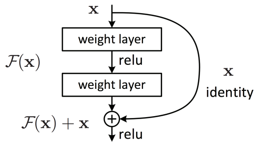
Fig. 2.13.: Illustration d'une couche résiduelle [He+16a]. L'entrée est additionnée aux résultats du mapping. Figure extraite du papier d'origine [He+16a]
