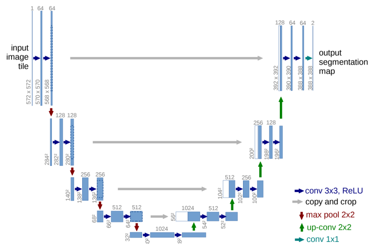
Fig. 4.15.: U-Net. Les cartes de caractéristiques extraites avant les opérateurs de sous-échantillonnage de la partie convolutive sont concaténées aux cartes de caractéristiques extraites après les opérateurs de sur-échantillonnage de la partie déconvolutive. Image tirée du papier [Ron+15].
