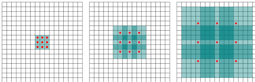
Fig. 4.17.: Champ réceptif des opérateurs de convolutions dilatées utilisant des facteurs de dilatations de 1, 2 et 4. Image tirée du papier [YK16].
