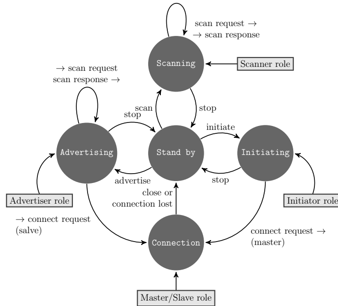
Figure 2.2: BLE Finite State Machine
