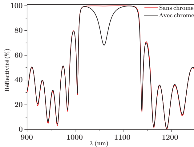
FIGURE 2.3 – Simulation de la réflectivité de Bragg HR avec et sans masque métallique pour le mode LG_{00} . Le calcul suppose un masque métallique de type croix simple (figure 2.2.a) d'épaisseur 5\text{ nm} et un miroir de Bragg de 27.5 paires. La longueur d'onde de travail est \lambda_0 = 1.060\text{ nm} .
