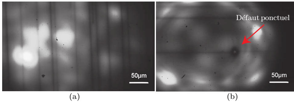
FIGURE 3.5 – Dislocation d'un échantillon comportant 24 puits quantiques InGaAs/GaAs. Bien que la contrainte de désaccord de maille soit compensée sur la totalité de la structure, l'utilisation de plusieurs puits par maximum de champ sur des longueurs réduites fragilise la structure et conduit finalement à sa relaxation.
