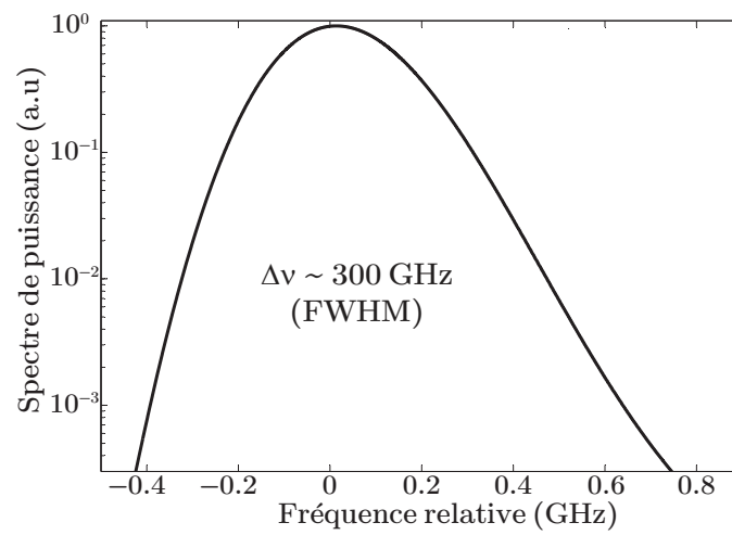
FIGURE 2.12 – Spectre mesuré et spectre simulé du VeCSEL sans mode à l'état stationnaire. On peut remarquer le caractère asymétrique du spectre à cause de décalage spectral introduit par l'AOM.
