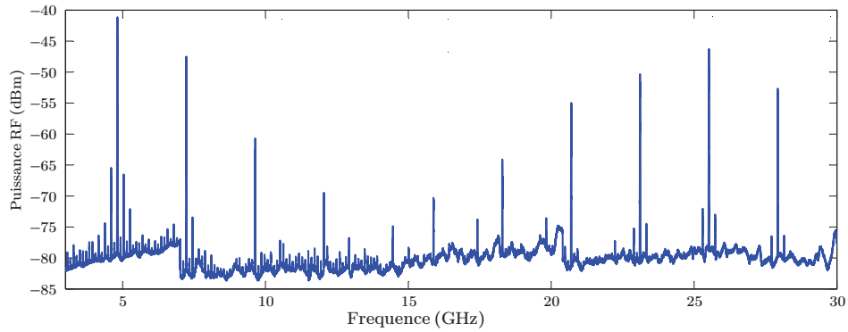
FIGURE 5.6 – Spectre RF du VeCSEL injecté par source mono-fréquence. La configuration de la cavité satisfait 1 \times f_s = 2 \times f_c avec f_c = 110 MHz . Le spectre RF ne correspond pas à un fonctionnement impulsionnel à 220MHz.
