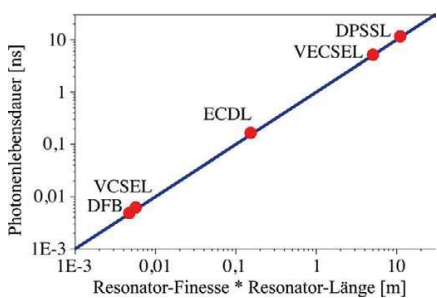
Bild 2: Photonenlebensdauer verschiedener Lasertechnologien: Mikroresonator-VCSEL, 300 µm DFB, 1 cm ECDL, 1 cm VeCSEL und 1 m Festkörperlaser (z.B. TiSa)
