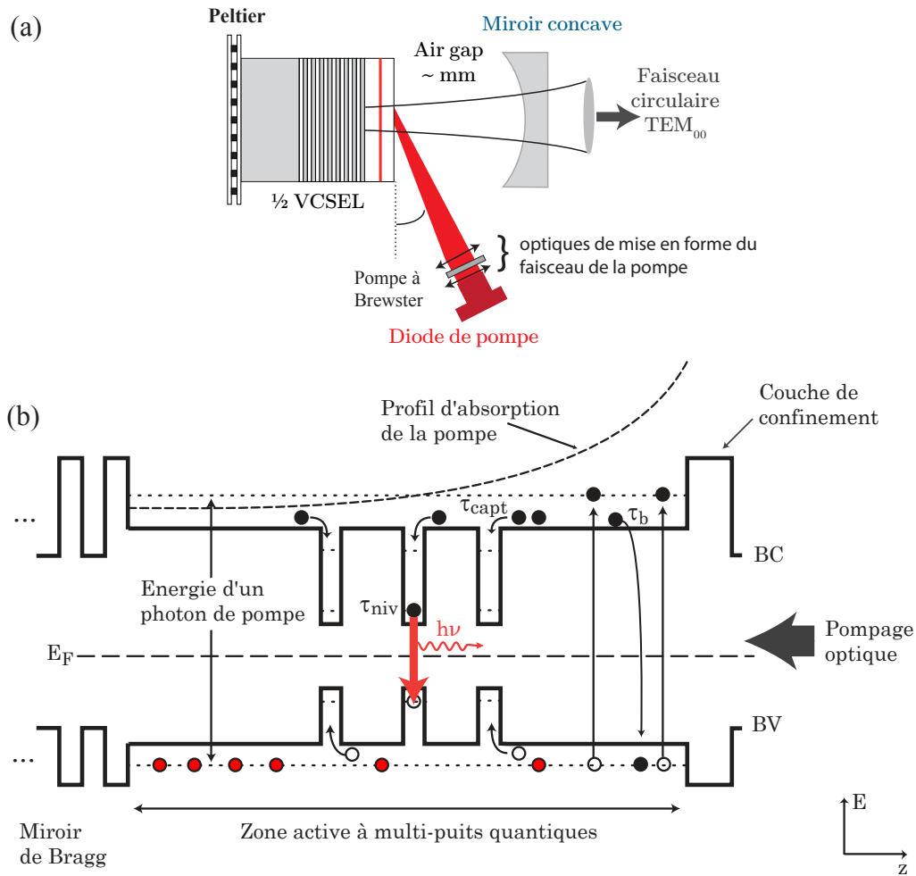
FIGURE 1.18 – a) Schéma de principe du pompage optique. b) Description schématique des différents processus intervenant dans une structure 1/2 VCSEL sous pompage optique. Les cercles noirs (blanc) représentent les états occupés par les électrons (trous).
