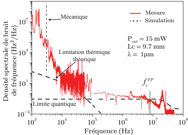
FIGURE 2.10 – Densité spectrale de bruit de fréquence de VeCSEL à 1\mu\text{m} . Les limitations théoriques de différentes origines sont indiquées. La limite théorique de bruit blanc a été calculée pour un facteur \alpha_h = 4 .
