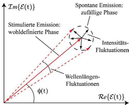
Bild 1: Das gesamte Laserfeld als Vektor-Konstruktion von spontaner Emission, die der stimulierten Emission überlagert ist
