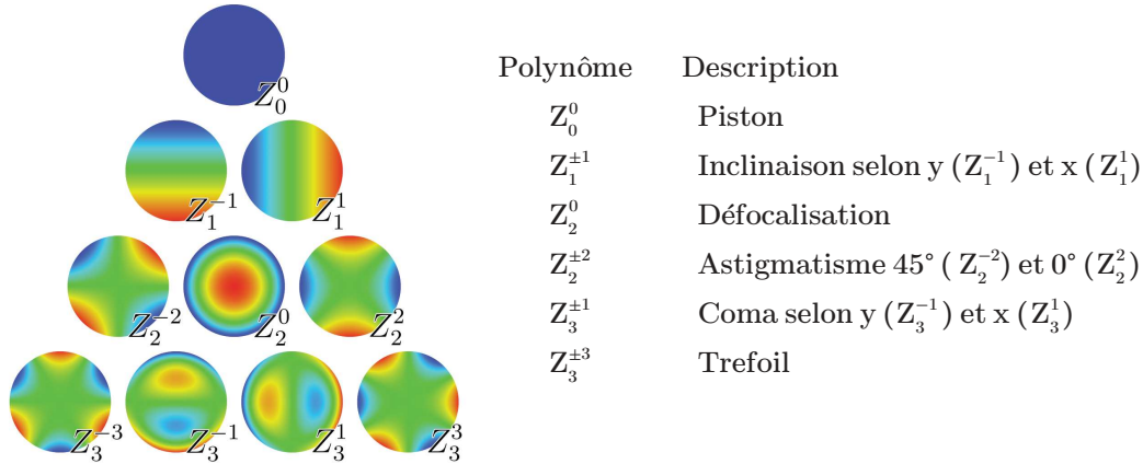
FIGURE 2.2 – Les premiers polynômes de Zernike
