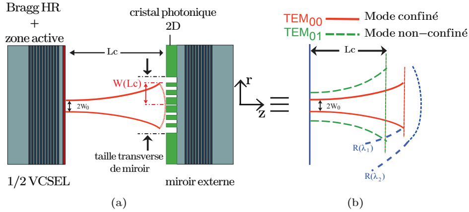
FIGURE 1.7 – a) Illustration schématique d'un VeCSEL avec un miroir externe à cristaux photonique. – b) Résonateur équivalent intrinsèquement monomode : la dépendance de réponse du cristal photonique en longueur d'onde introduit naturellement un filtrage spectral. D'après [Seghilani 2014].
