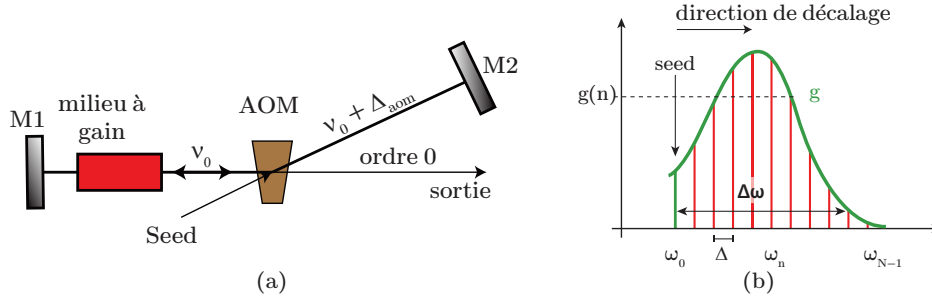
FIGURE 5.1 – a) Illustration schématique d'un laser FSF injecté par un laser monofréquence. b) Le spectre optique du laser FSF injecté consiste en un peigne de fréquences espacé de la fréquence de décalage \Delta_{aom} .
