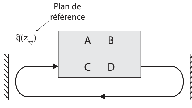
FIGURE 1.20 – Illustration du modèle de calcul de la stabilité d'une cavité optique. La cavité est stable si \tilde{q}(z) n'est pas changé après un aller-retour dans la cavité.
