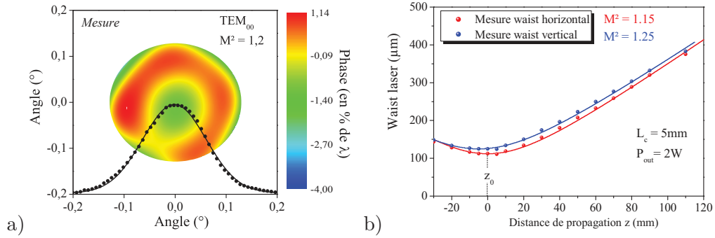
FIGURE 2.3 – a) Mesure de front d'onde en champ lointain à forte puissance (2.1W) pour un VeCSEL émettant à 1µm. Le rayon de courbure de champ a été retiré.– b) Mesures expérimentales et simulations de l'évolution de la taille du waist laser en fonction de la distance de propagation pour les deux axes du faisceau. d'après[Laurain 2010b].
