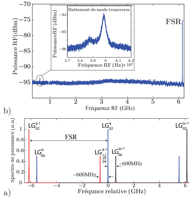
FIGURE 3.5 – a) Mesure du spectre radio fréquence de bruit d'intensité de VeCSEL à 1\ \mu\text{m} , émettant sur le mode transverse LG_{02} dégénéré, sur une gamme de fréquences allant jusqu'au premier harmonique des battements des modes longitudinaux. En zoom, le signal de battement dû aux modes transverses faibles (résolution 20 kHz). — b) Spectre théorique de la cavité froide du VeCSEL.
