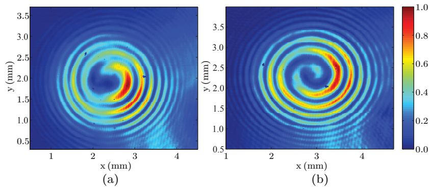
FIGURE 3.7 – Mode LG 01 vortex contrôlé en signe de charge topologique avec un masque de phase perturbatif. Le signe de la charge suit le sens croissant de la phase induite par le cristal photonique. —a) m = -1 . —b) m = +1 .
