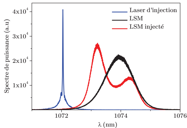
FIGURE 5.4 – Spectre optique du VeCSEL FSF. En noir : Spectre du laser en régime FSF sans mode ( \sim 300 GHz FWHM). En rouge : Spectre du laser injecté. En bleu : Spectre de laser d'injection.
