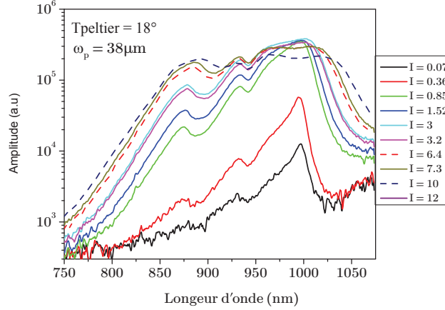
FIGURE 3.6 – Spectre de photoluminescence observé par la tranche d'une structure 1/2 VCSEL à 12 puits quantique en GaAs émettant à 1\mu\text{m} . Les densités d'excitation I sont en \text{kW}/\text{cm}^2 .
