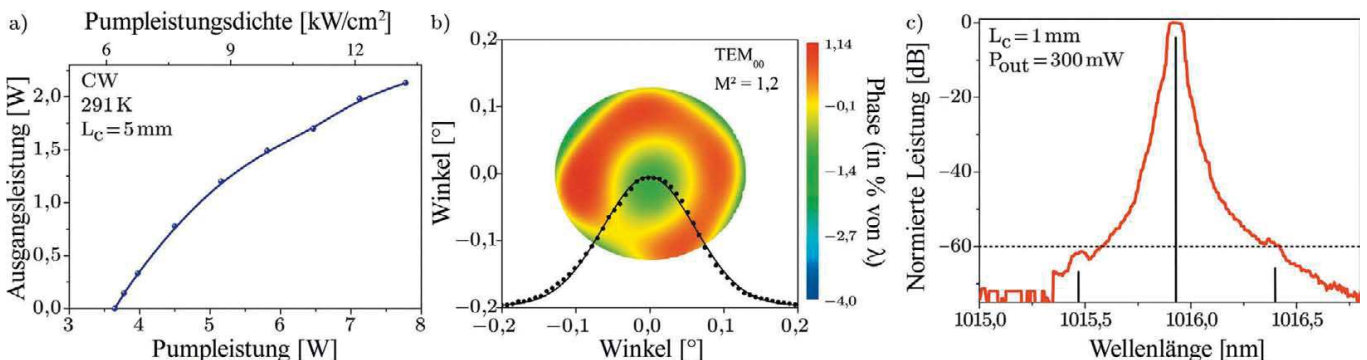
Bild 4: Haupteigenschaften von OP-VeCSELn, a) mehrere Watt Ausgangsleistung, b) TEM 00 beugungsbegrenzter Strahl (Phasenvariation < \lambda/100 ), c) Einzelfrequenzbetrieb mit hoher SMSR
