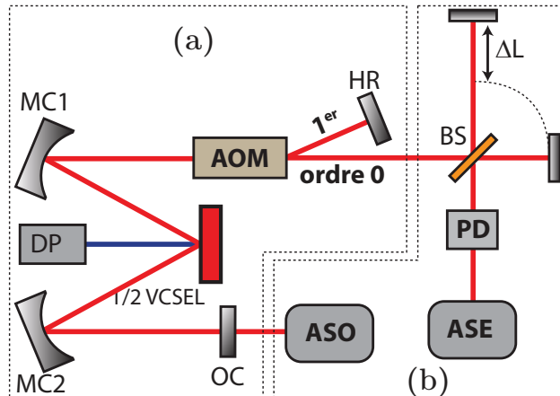
FIGURE 4.4 – Montage expérimental pour la caractérisation du VCSEL sans mode. –a) laser sans mode. MC miroir concave; DP diode de pompe. –b); ASO Analyseur de spectre optique; ASE analyseur de spectre électrique; BS : beam splitter; PD photodiode.
