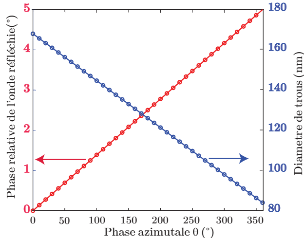
FIGURE 2.11 – Graphe de conception de la dépendance spatiale de la taille des trous pour réaliser une fonction de perturbation de phase azimutale. Pour le calcul, on considère une structure anti-résonante et une épaisseur de \text{Si}_3\text{N}_4 de 75 \text{ nm} . La période du cristal photonique est de 280 \text{ nm} et ff \in [0.3 \ 0.6] .
