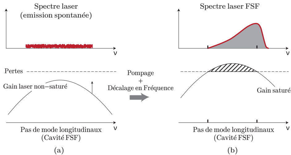
FIGURE 2.2 – Illustration schématique du processus de saturation du gain dans un laser FSF. –a) Lorsque le gain < pertes optiques, la sortie du FSF est juste le bruit d'émission spontanée. –b) Après saturation : la saturation du gain est fixée par un équilibre entre l'affinement spectral dû à la courbure de gain et l'étalement spectral dû au décalage en fréquence. Le gain est saturé par une intensité totale répartie sur une plage spectrale large.
