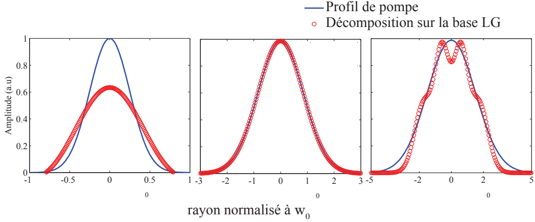
FIGURE 1.13 – Exactitude de la décomposition d'une pompe gaussienne sur la base de modes LG. De gauche à droite : w_p/w_0 = 0.5, 1.7 et 3 .
