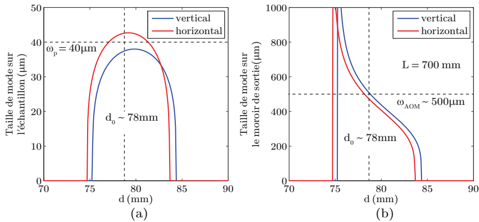
FIGURE 3.11 – Calcul de stabilité de la cavité linéaire. Le point de fonctionnement d_0 (voir figure 3.10) est choisi pour optimiser à la fois le recouvrement avec la pompe et l'efficacité de l'AOM.
