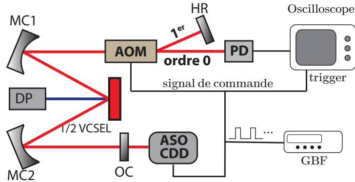
FIGURE 4.9 – Montage expérimental pour l’observation du démarrage et l’évolution de spectre optique de VeCSEL sans mode. Le rapport cyclique du signal de commande est ajusté pour permettre l’observation de l’évolution du spectre du laser dans une fenêtre temporelle au cours de démarrage du laser. Le temps de réponse de l’AOM est suffisamment court pour ne pas influencer la dynamique laser.
