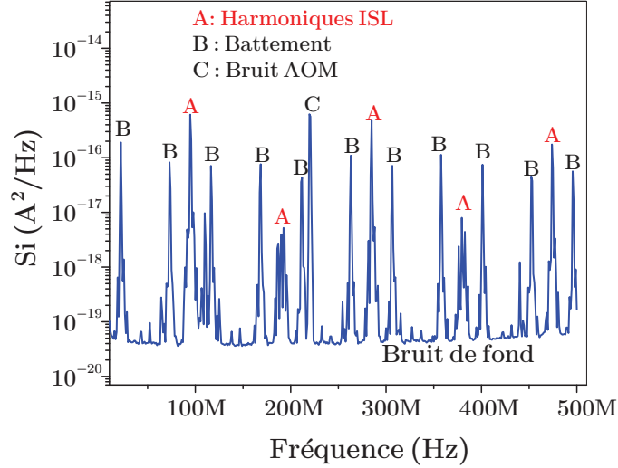
FIGURE 4.7 – Spectre RF du bruit d'intensité du laser sans mode à la sortie de l'interféromètre de Michelson. Pour cette mesure, la différence de marche est de \sim 30\text{cm} , équivalente à un décalage de fréquence de f_b \sim 21\text{ MHz} . Les battements à la fréquence f_b et q \times ISL \pm f_b qui apparaissent sur le spectre RF de bruit sont caractéristiques des lasers sans mode et peuvent être utilisées dans les mesures de distance.
