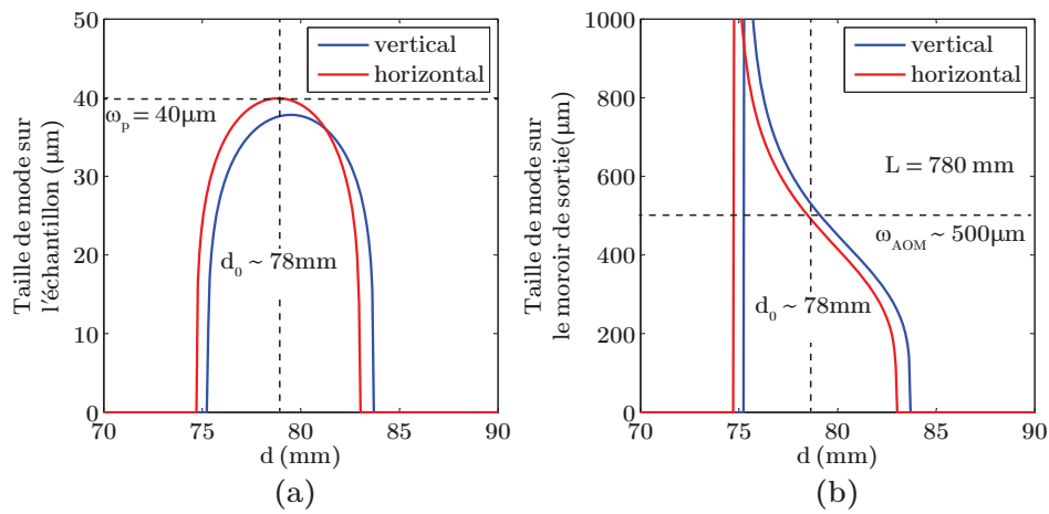
FIGURE 3.12 – Calcul de stabilité de la cavité linéaire. Le point de fonctionnement d_0 (voir figure 3.10) est choisi pour optimiser à la fois le recouvrement avec la pompe et l'efficacité de l'AOM.
