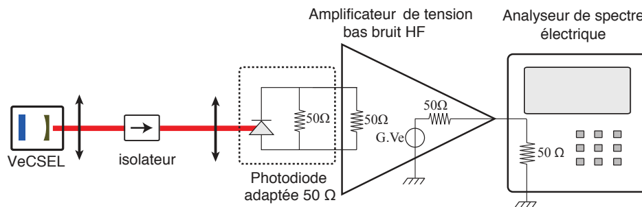
FIGURE 2.5 – Montage expérimental pour la mesure du bruit d'intensité à haute fréquence.
