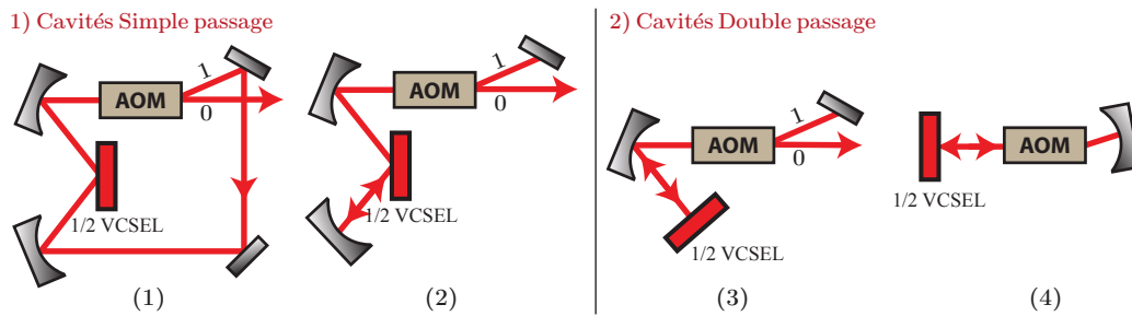
FIGURE 3.9 – Variantes de cavités optiques possibles pour un laser sans mode VCSEL. (1) cavité en anneau. (2) cavité linéaire avec double passage dans la zone active. (3)(4) Cavité linéaire, avec (4) une version très compacte limitée essentiellement par la taille de l'AOM.
