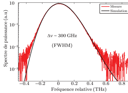
FIGURE 4.3 – Spectre optique du VeCSEL sans mode émettant autour de 1.07\mu\text{m} : la largeur à mi-hauteur et de \sim 300 GHz ( \sim 1.15 ).
