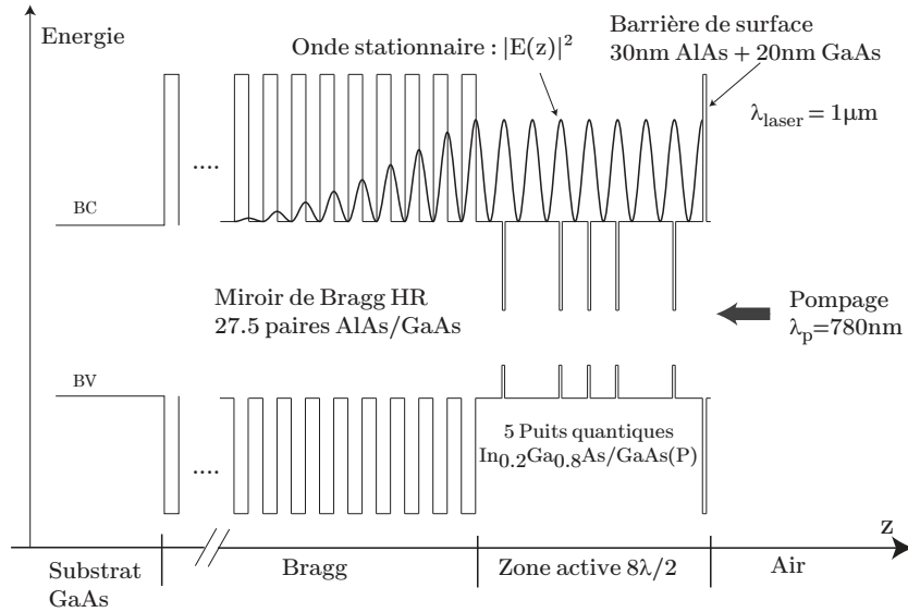
FIGURE 2.1 – Diagramme d'énergie de la structure 1/2 VCSEL émettant à 1\mu m . La structure est en configuration de micro cavité résonante L_{za} = 8\lambda/2 .
