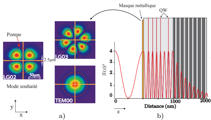
FIGURE 2.2 – Masque métallique en chrome déposé sur une structure résonante. a) plan transverse montrant le recouvrement d'un masque en croix simple pour le mode LG_{02} avec les modes non-souhaités. b) position du masque sur un ventre de champ dans la direction de croissance pour maximiser l'absorption.
