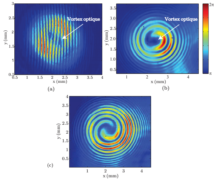
FIGURE 3.6 – Signature de la singularité de phase des modes LG 01 et LG 02 vortex. — a) Interférence en champ proche avec une onde de référence plane. La charge topologique du vortex est la différence du nombre de franges de part et d’autre de la singularité de phase, et son signe est la direction de la fourche. — b) Interférence en champ proche avec une onde de référence sphérique. Ici la charge topologique du vortex est le nombre de spirales, et son signe est la direction de rotation de la spirale. Ici on a m = -1 . — c) Mode vortex LG 02
