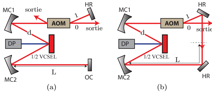
FIGURE 3.10 – Illustration schématique de la cavité optique du VeCSEL sans mode à 1\mu\text{m} . — a) Configuration de cavité linéaire en M. — b) Configuration de cavité en anneau. Les longueurs L et d intervenant dans le calcul de stabilité sont aussi présentées. DP : diode de pompe ; MC : miroir concave de repli ; AOM : modulateur acousto-optique ; HR : miroir de haute réflectivité ; OC : coupleur
