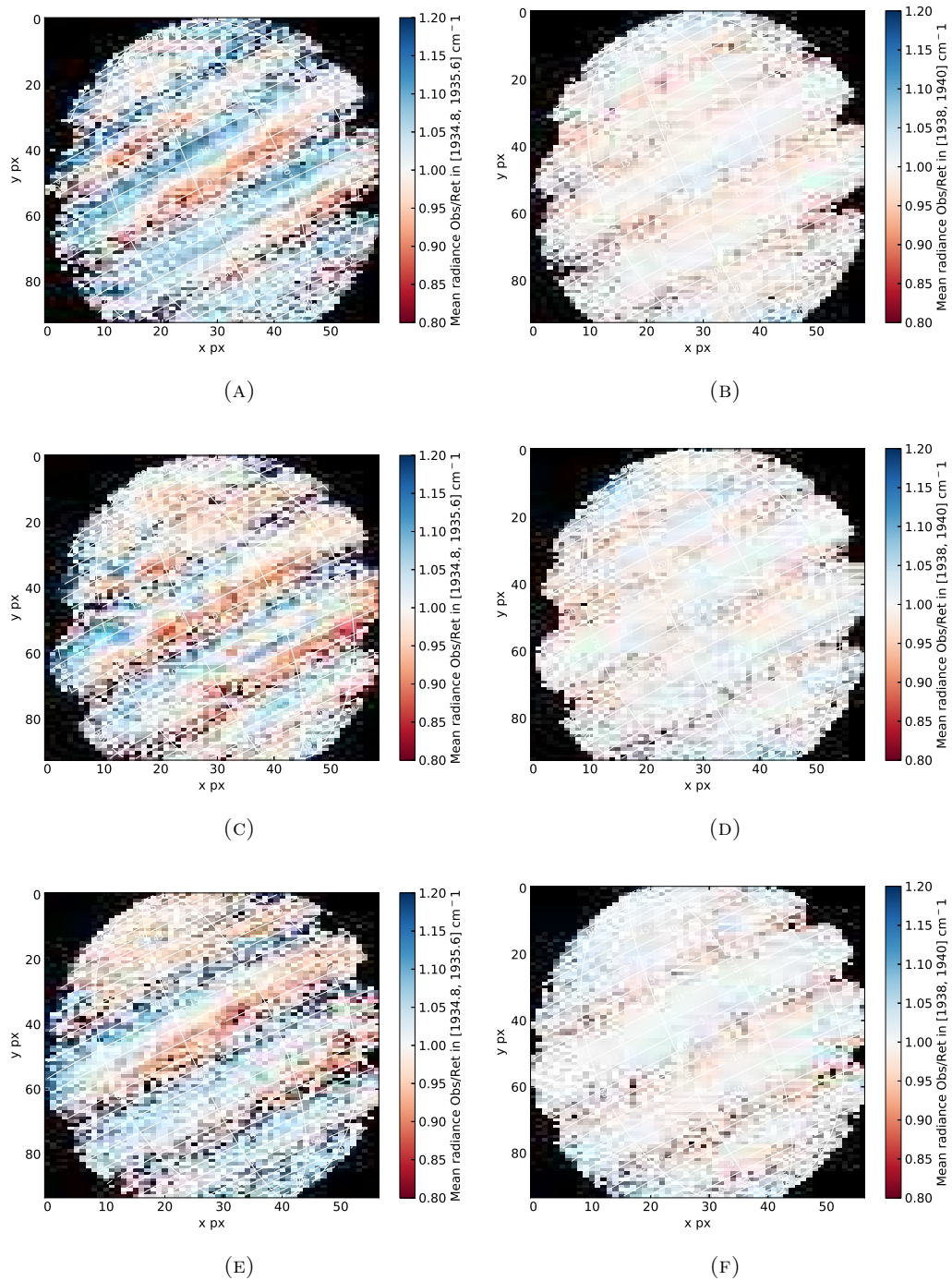
FIGURE 4.15 – Exemple de carte de structure spectrale inexplicée, sur les trois cubes spectraux analysés. De haut en bas : cubes spectraux SC1, SC2 et SC3. Gauche : rapport, entre 1934.8 et 1935.6 \text{cm}^{-1} , de la moyenne des radiances observée sur la moyenne des radiances du spectre synthétique ajusté. Droite : rapport, entre 1938 et 1940 \text{cm}^{-1} (où se trouve la raie principale de \text{NH}_3 ), de la moyenne des radiances observée sur la moyenne des radiances du spectre synthétique ajusté.
