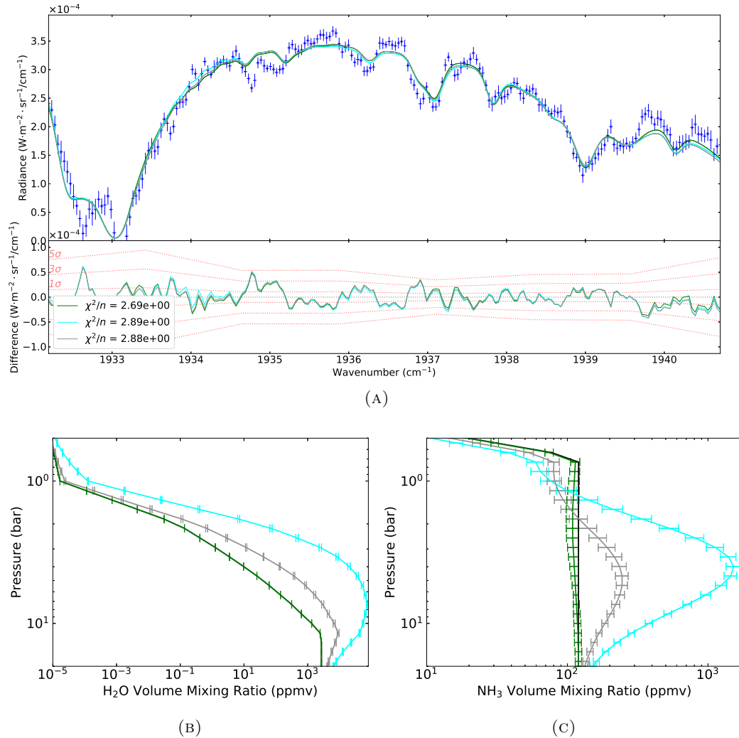
FIGURE 4.11 – Influence de l'H 2 O sur l'inversion. Bleu foncé : spectre observé. Vert : spectre (figure du haut), profil d'abondance de l'H 2 O (figure en bas à gauche) et profil d'abondance du NH 3 (figure en bas à droite) obtenus en inversant la transmittance du nuage (valeur obtenue : 0,131) et le profil d'abondance de NH 3 , mais en gardant le profil d'abondance de l'H 2 O constant. Bleu clair : idem, mais le profil d'abondance de l'H 2 O est inversé, tandis que la transmittance du nuage est fixée à 1. Gris : idem, mais les deux profils d'abondances moléculaires sont inversés en même temps que la transmittance du nuage (valeur obtenue : 0,248). Noir : profil d'abondance a priori du NH 3 utilisé pour inverser le spectre observé. Le résidu de ces spectres par rapport au spectre observé est représenté dans la partie basse de la figure du haut.
