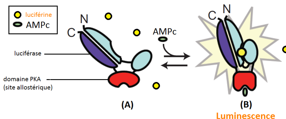
Figure 14 : Fonctionnement du GloSensor (Fan et al., 2008). Une sous-unité régulatrice de la PKA est insérée dans la luciférase et régule son activité (luminescence) de manière allostérique sous la dépendance de l'AMPc. Conformation inactive (A) et active (B) de la luciférase dite Glosensor.
