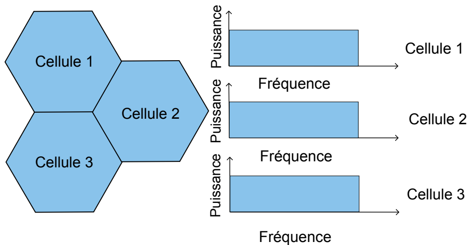
FIGURE 1.2 – L'approche Reuse 1.
