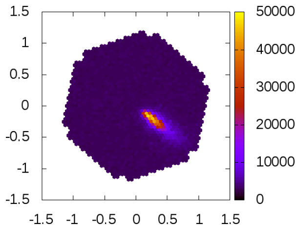
FIGURE 4.9 – Illustration de la forme ellipsoïdale des gerbes enregistrées dans les caméras des simulations Monte-Carlo. L'échelle de couleurs représente le nombre de photons détectés dans un pixel.
