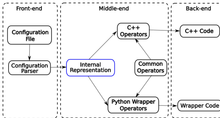
FIGURE 3.9 – Illustration de l'architecture de la deuxième version du générateur de formats de données.
